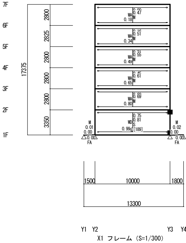
終局時機構図（Y方向 負加力）（立体MSモデル）（保有耐力時）
