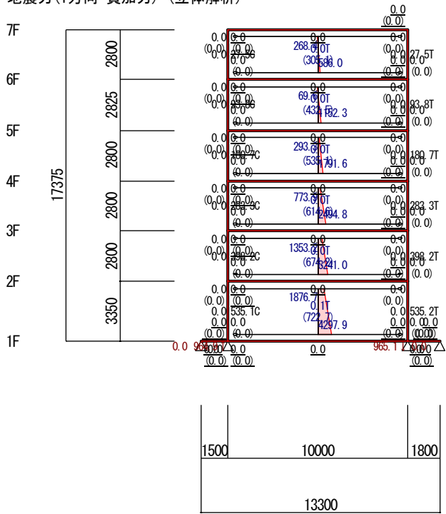
地震力 (Y方向 負加力) (立体解析)
