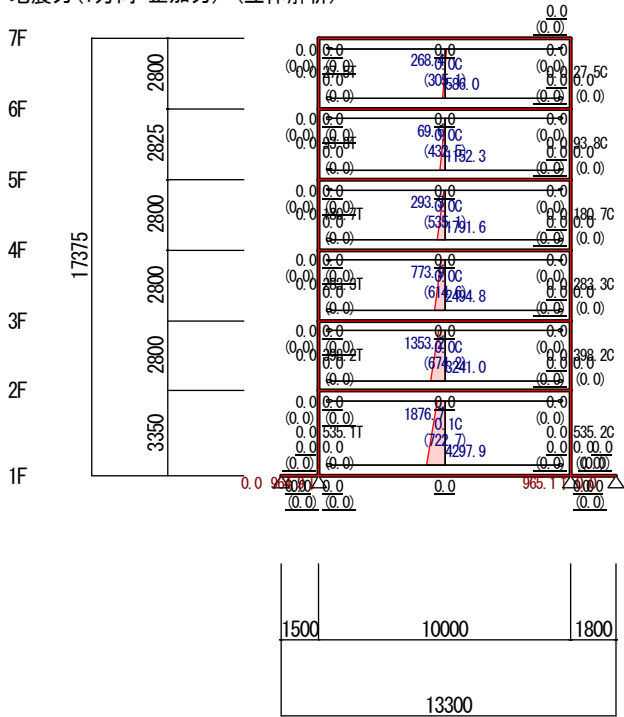
地震力(Y方向 正加力) (立体解析)
