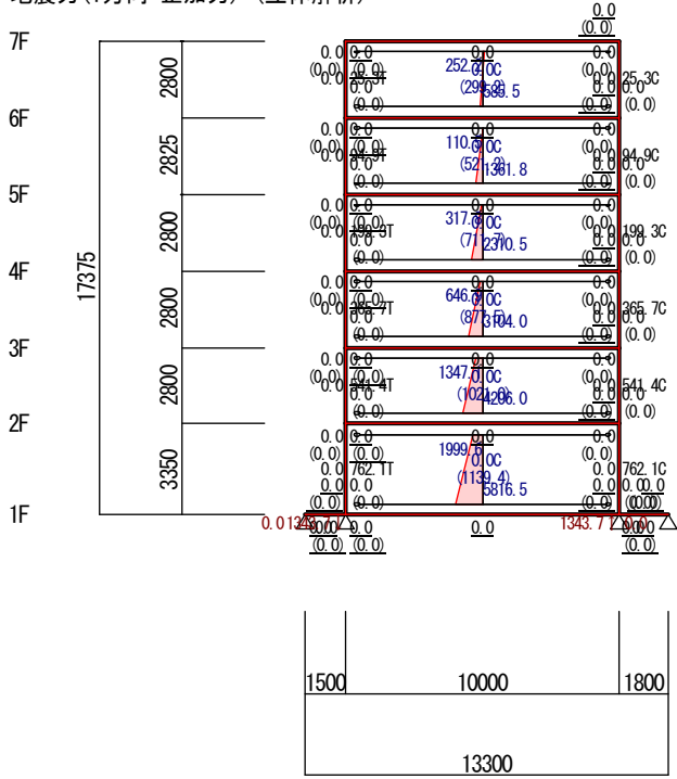
地震力(Y方向 正加力) (立体解析)
