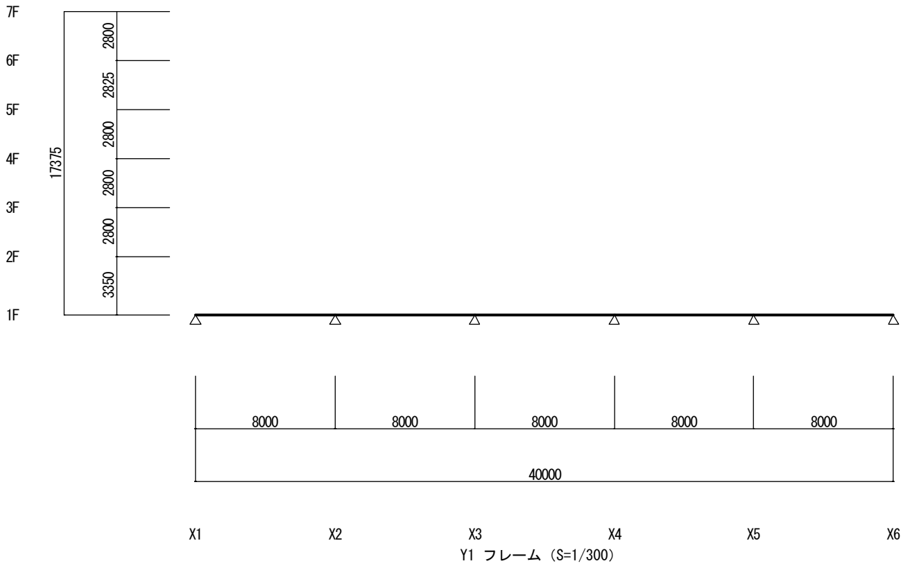
ヒンジ図（X方向 負加力）（立体MSモデル）（Ds算定時）
