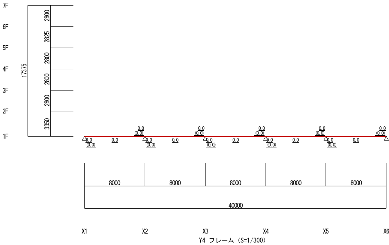
水平荷重時節点応力（X方向 負加力）（立体MSモデル）（保有耐力時）
