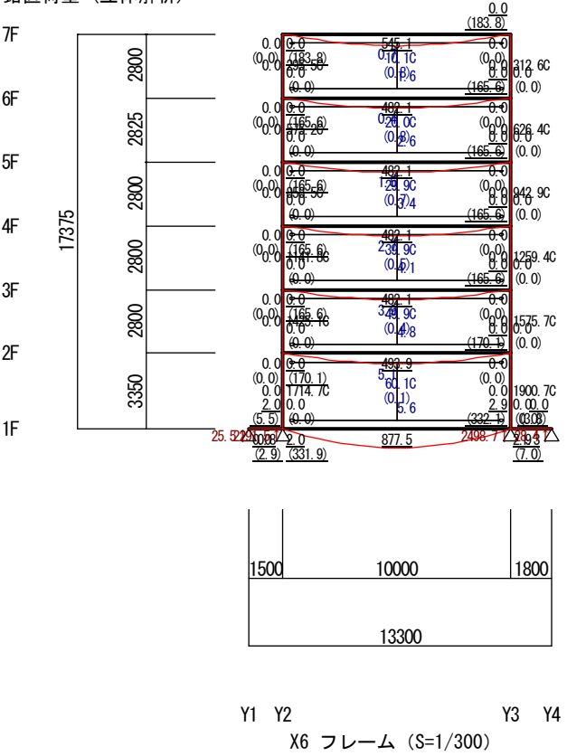
鉛直荷重 (立体解析)
