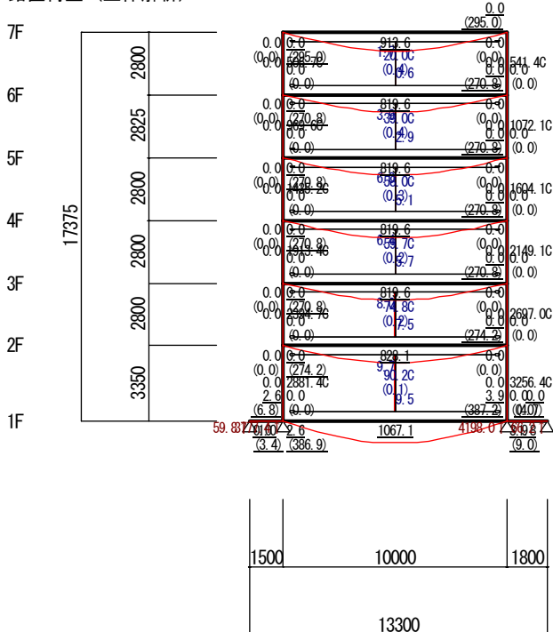
鉛直荷重 (立体解析)
