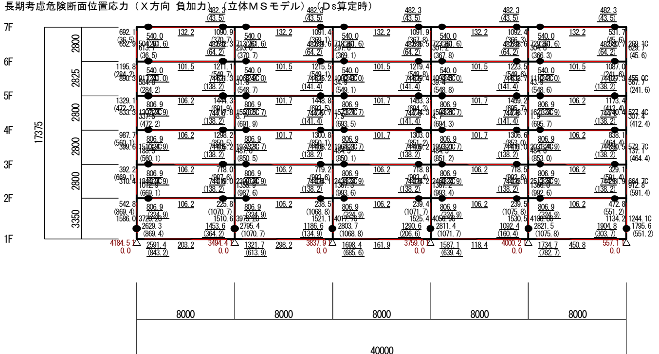
長期考慮危険断面位置応力 (X方向 負加力) (立体MSモデル) (Ds算定時)
