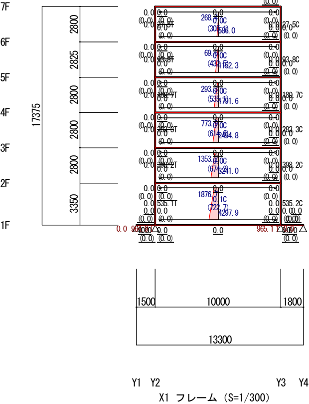
地震力(Y方向 正加力) (立体解析)
