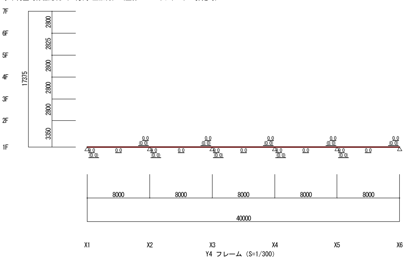
水平荷重時節点応力 (X方向 正加力) (立体MSモデル) (Ds算定時)
