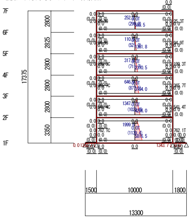
地震力 (Y方向 負加力) (立体解析)
