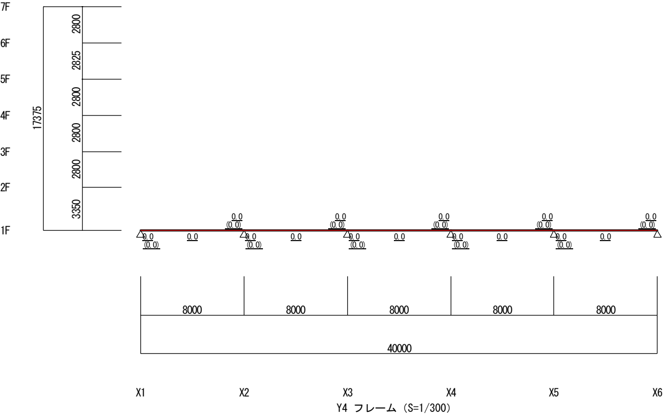
水平荷重時節点応力（X方向 正加力）（立体MSモデル）（保有耐力時）
