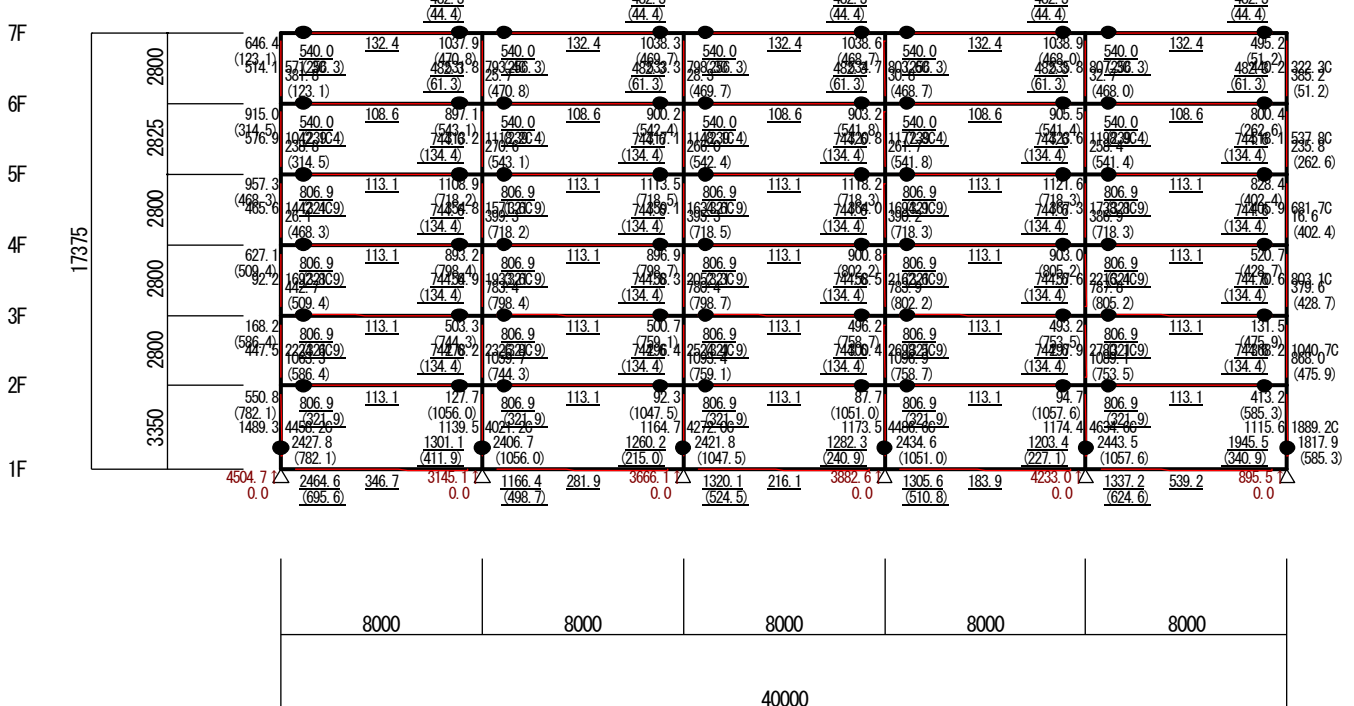
長期考慮危険断面位置応力 (X方向 負加力) (立体MSモデル) (Ds算定時)
