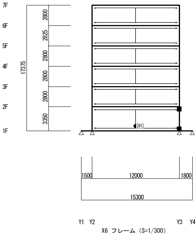
ヒンジ図 (Y方向 負加力) (立体MSモデル) (Ds算定時)
