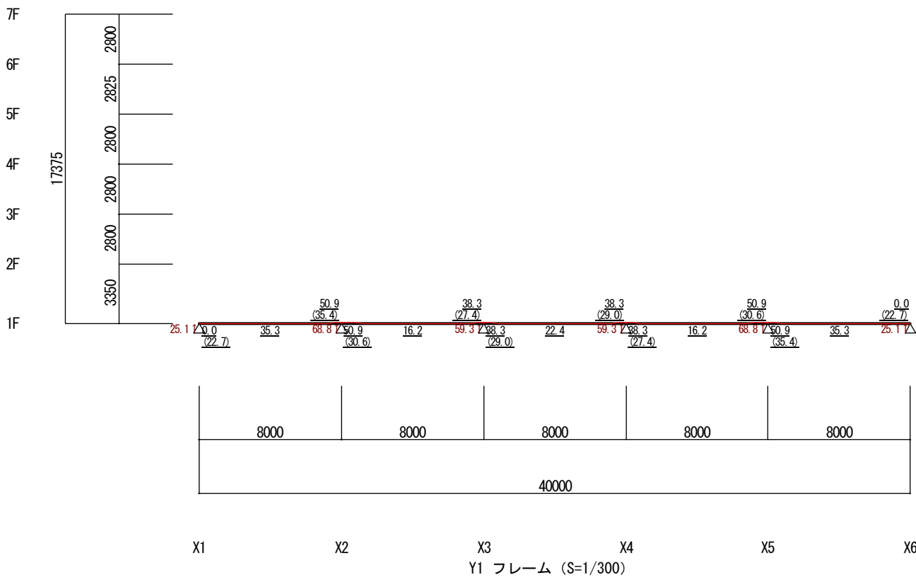
鉛直荷重（立体解析）
