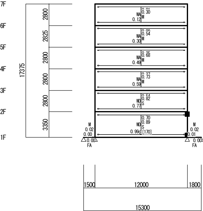
終局時機構図（Y方向 負加力）（立体MSモデル）（保有耐力時）
