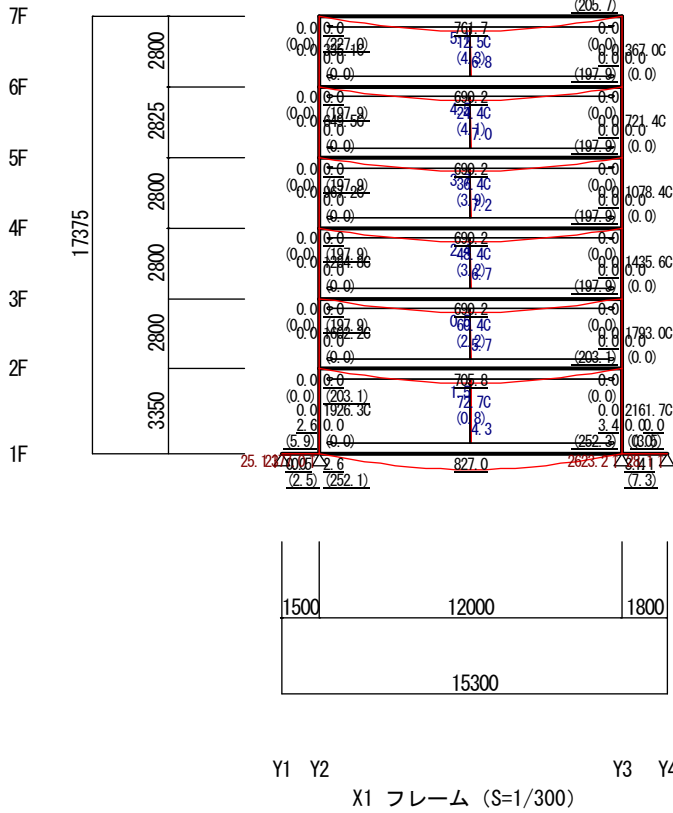
鉛直荷重 (立体解析)
