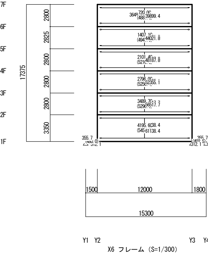
終局強度（Ｙ方向 負加力）（立体MSモデル）（Ds算定時）
