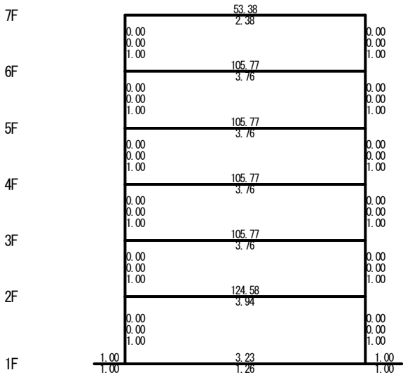
X1 X2 X3 X4 X5 X6 Y4 フレーム (S=1/263)
