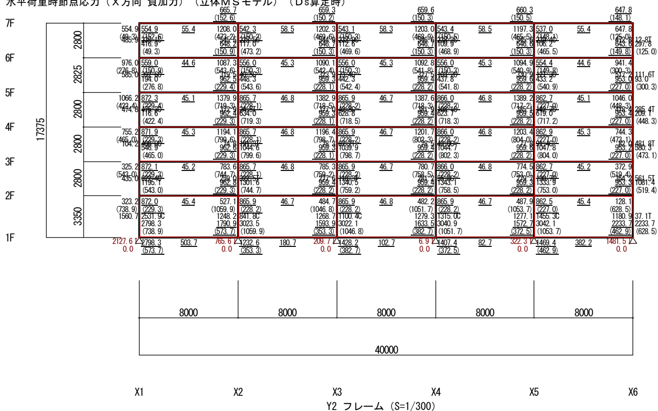
水平荷重時節点応力 (X方向 負加力) (立体MSモデル) (Ds算定時)
