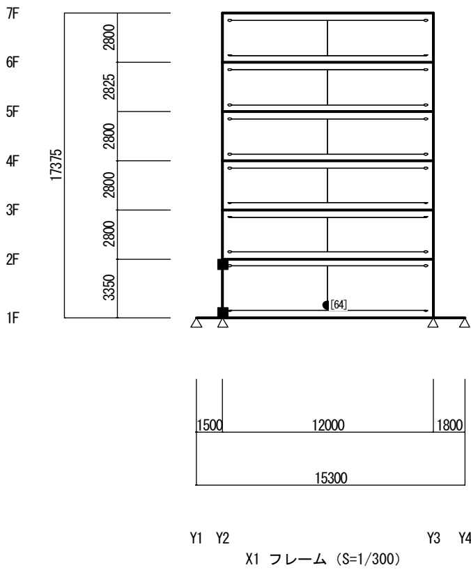
ヒンジ図（Y方向 正加力）（立体MSモデル）（Ds算定時）
