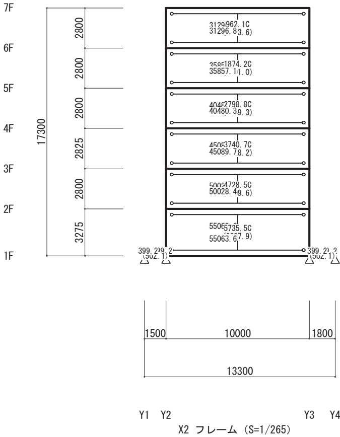
終局強度（Ｙ方向 正加力）（立体MSモデル）（Ds算定時）
