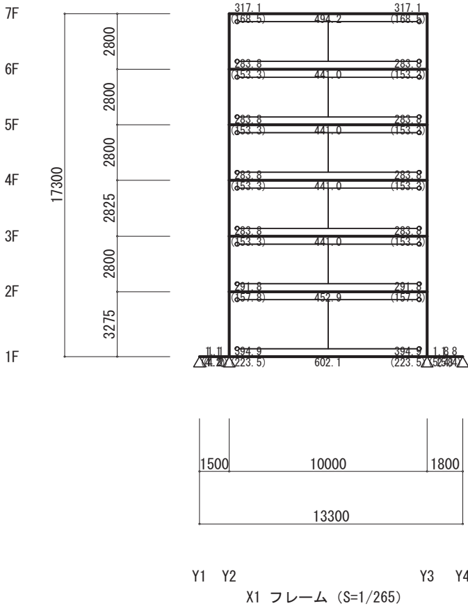
固定荷重＋積載荷重
