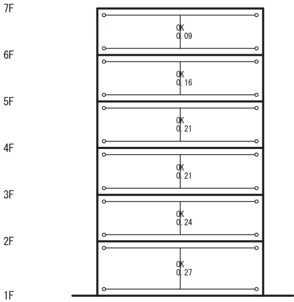
Y1 Y2 Y3 Y4 X1 フレーム (S=1/233)
