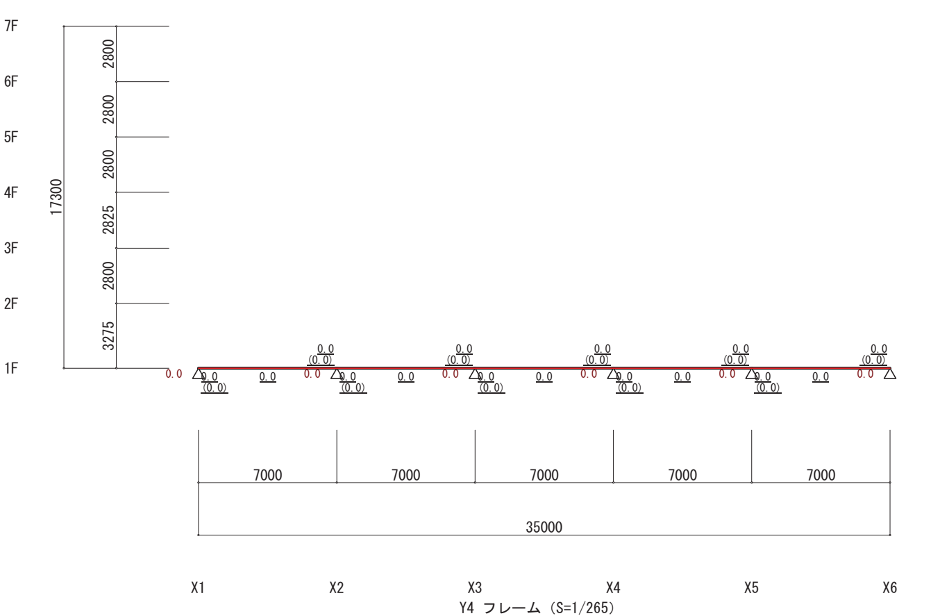
地震力(X方向 負加力) (立体解析)
