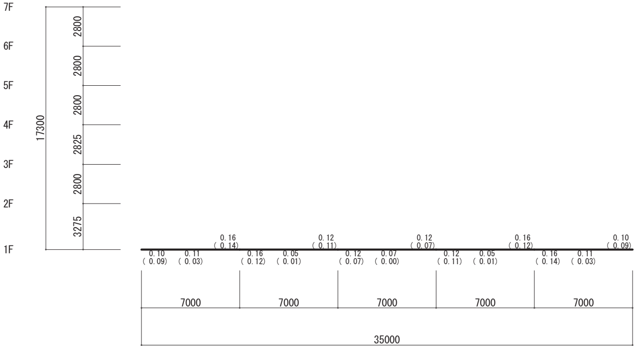
X1 X2 X3 X4 X5 X6 Y4 フレーム (S=1/265)
