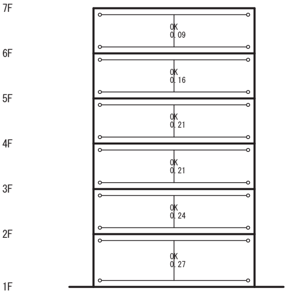
Y1 Y2 Y3 Y4 X2 フレーム (S=1/233)
