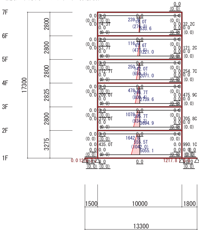
地震力(Y方向 正加力) (立体解析)
