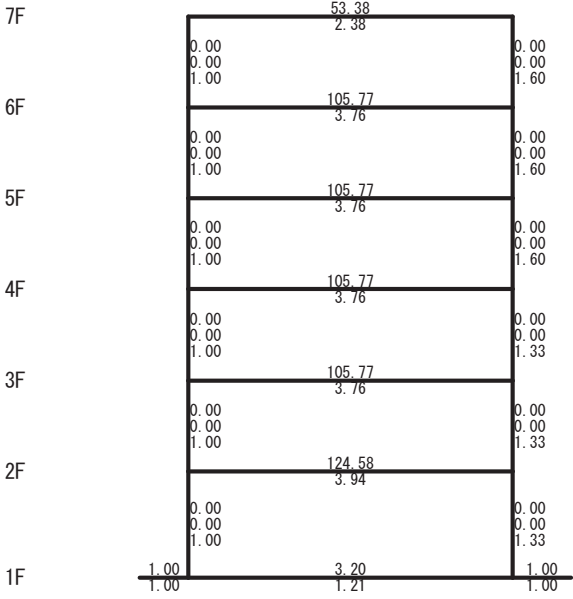
Y1 Y2 Y3 Y4 X2 フレーム (S=1/233)
