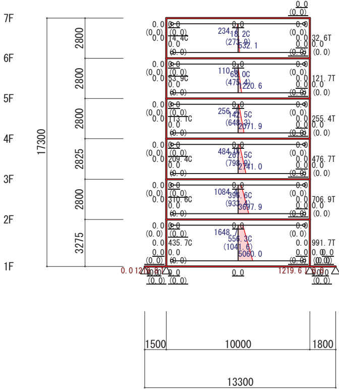
地震力(Y方向 負加力) (立体解析)
