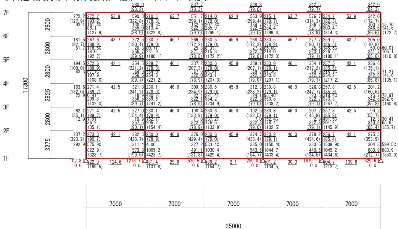
水平荷重時節点応力 (X方向 負加力) (立体MSモデル) (Ds算定時)
