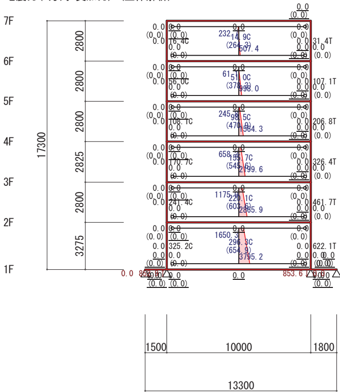
地震力 (Y方向 負加力) (立体解析)
