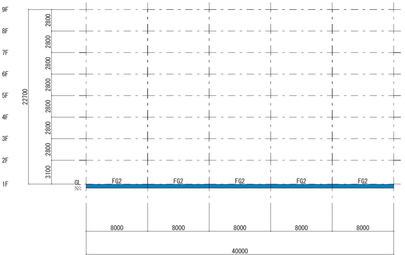
X1 X2 X3 X4 X5 X6 Y4 フレーム (S=1/300)
