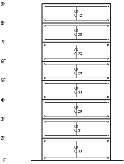
Y1 Y2 Y3 Y4 X2 フレーム (S=1/263)
