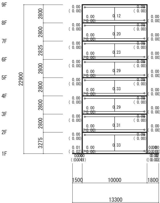
Y1 Y2 Y3 Y4 X2 フレーム (S=1/300)
