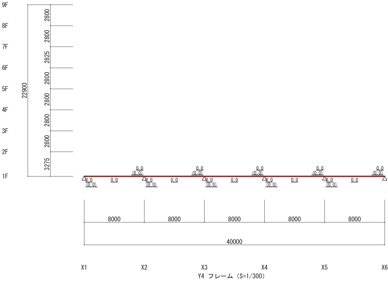
水平荷重時節点応力（X方向 正加力）（立体MSモデル）（保有耐力時）
