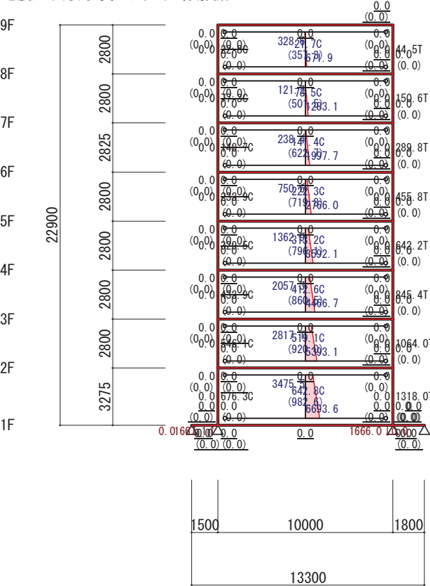
地震力(Y方向 負加力) (立体解析)
