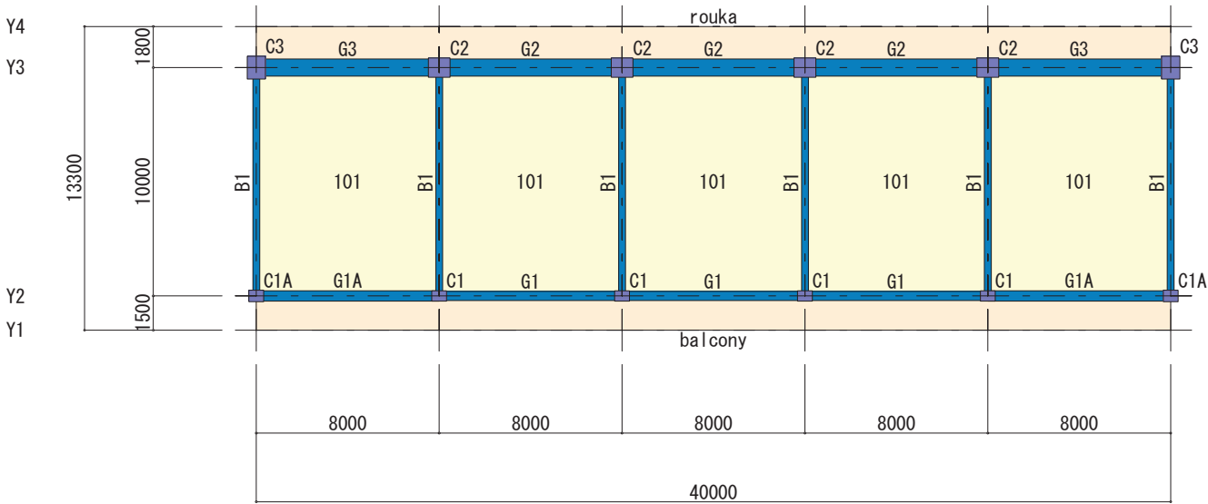
4F 層 (S=1/300)
