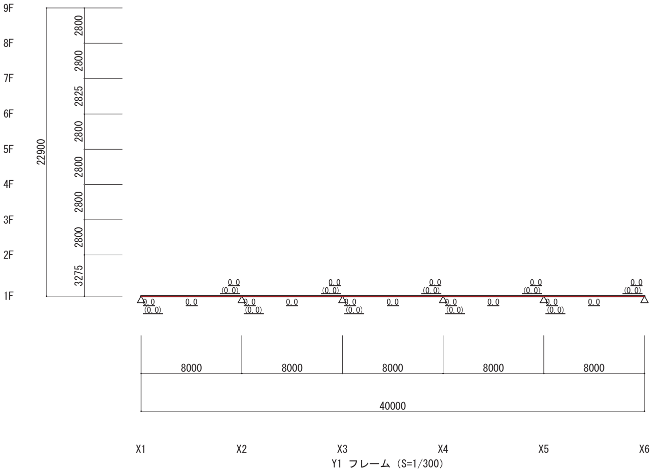
水平荷重時節点応力（X方向 負加力）（立体MSモデル）（Ds算定時）
