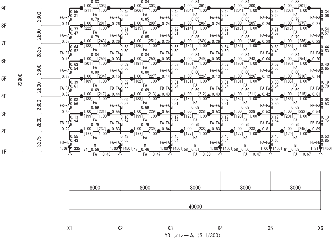
終局時機構図 (X方向 正加力) (立体MSモデル) (保有耐力時)
