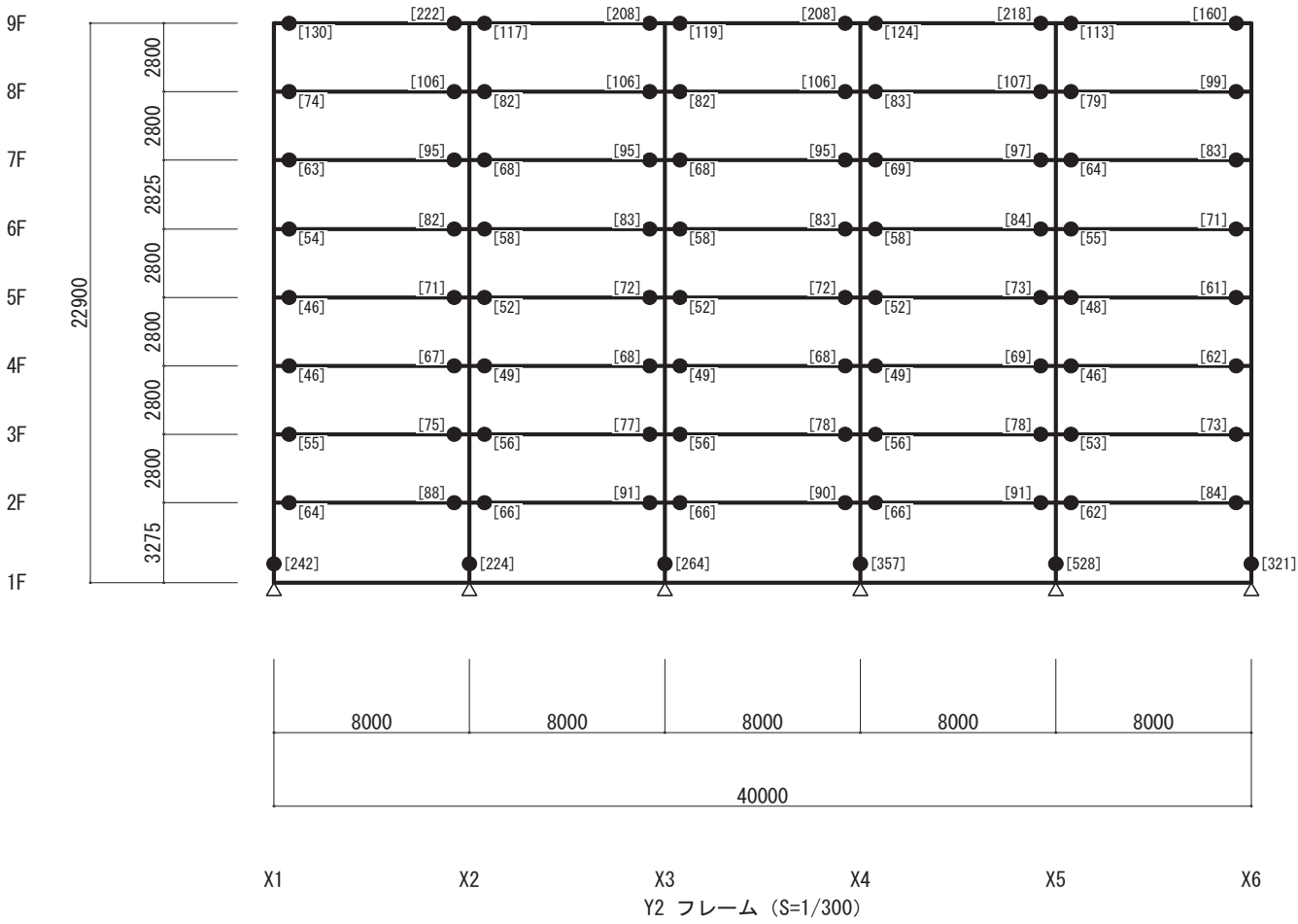
ヒンジ図 (X方向 負加力) (立体MSモデル) (Ds算定時)
