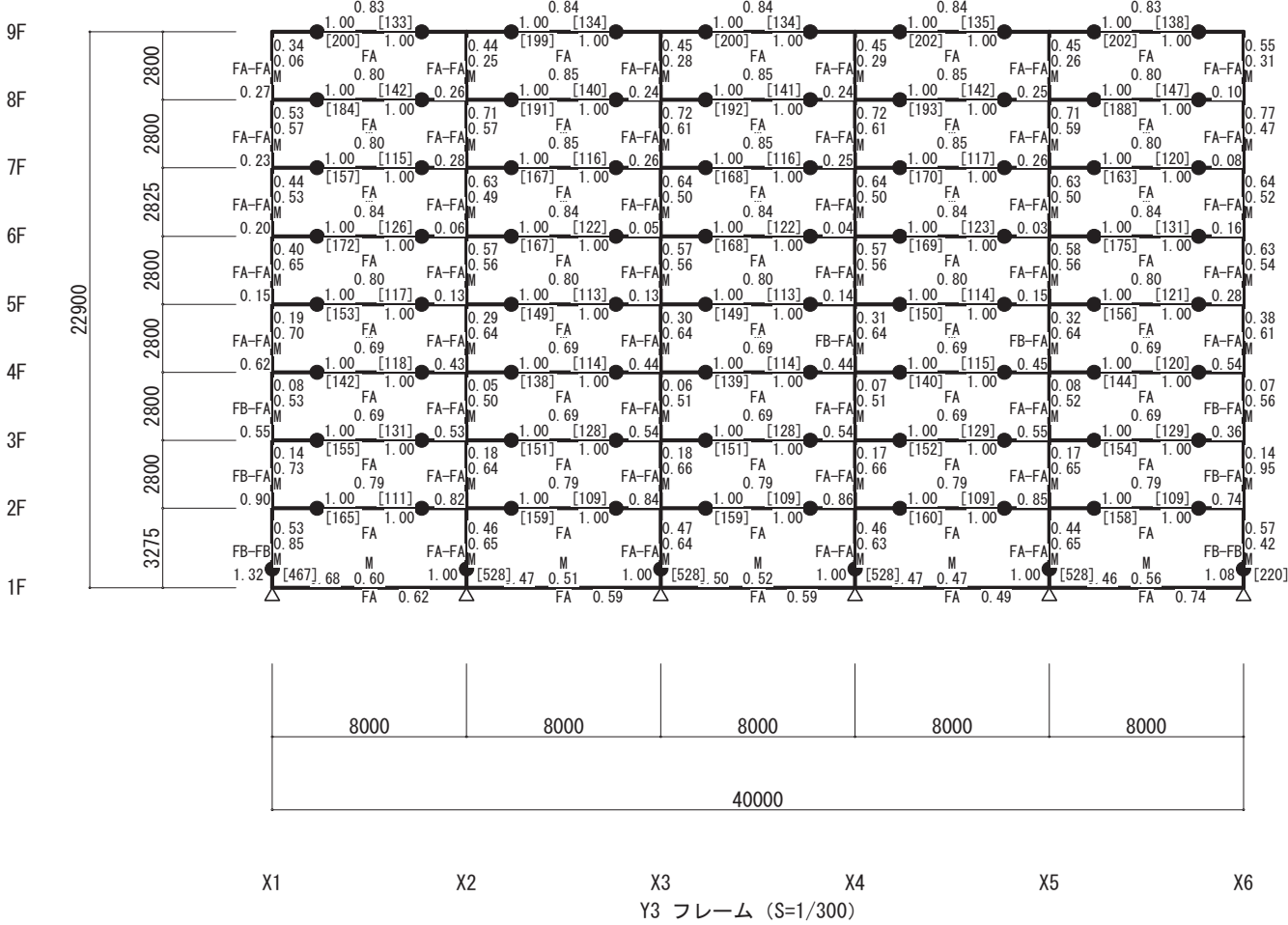
終局時機構図 (X方向 負加力) (立体MSモデル) (Ds算定時)
