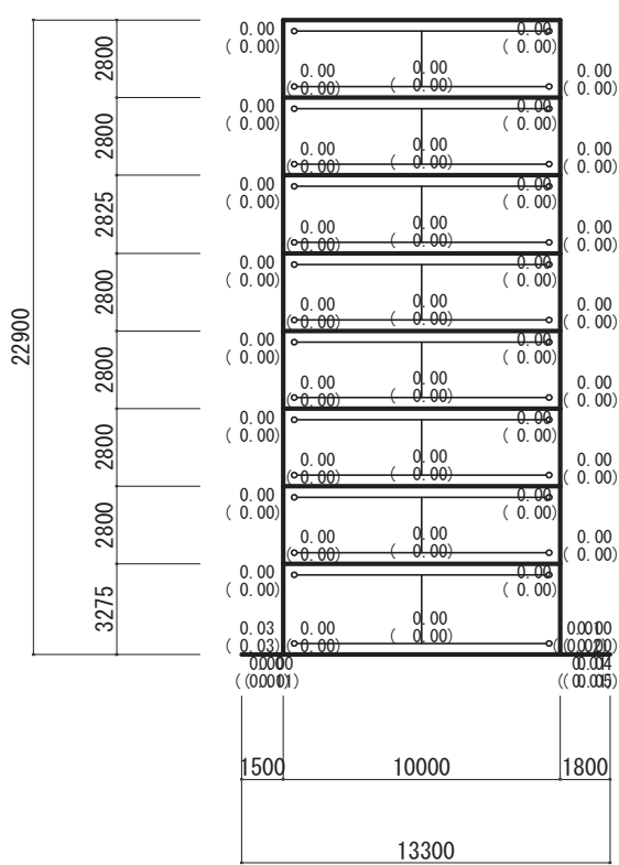
Y1 Y2 Y3 Y4 X2 フレーム (S=1/300)
