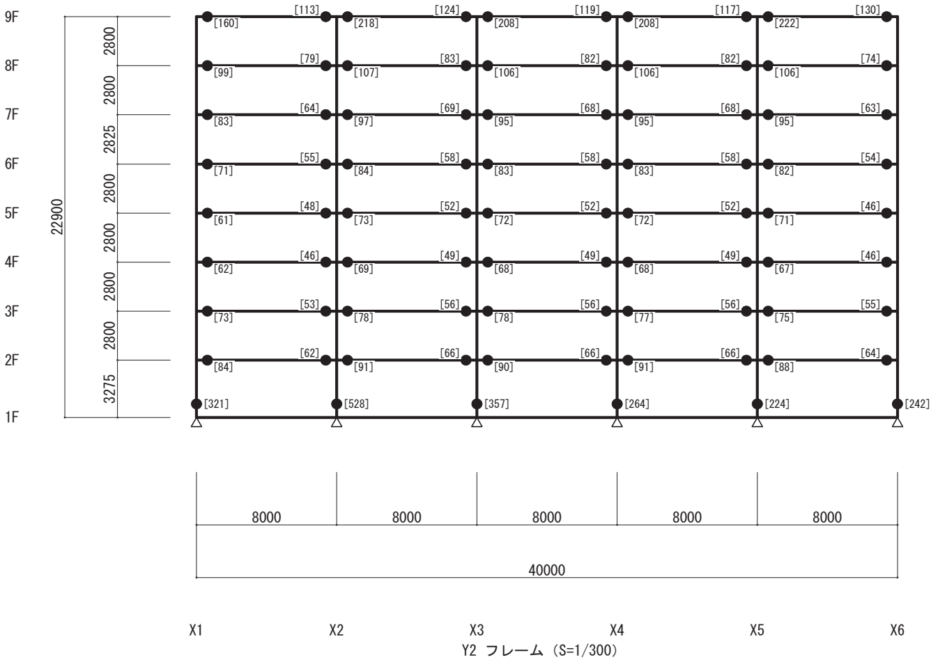
ヒンジ図 (X方向 正加力) (立体MSモデル) (Ds算定時)
