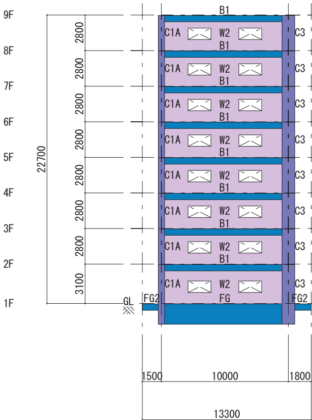
X1 X2 X3 X4 X5 X6 Y4 フレーム (S=1/300)
