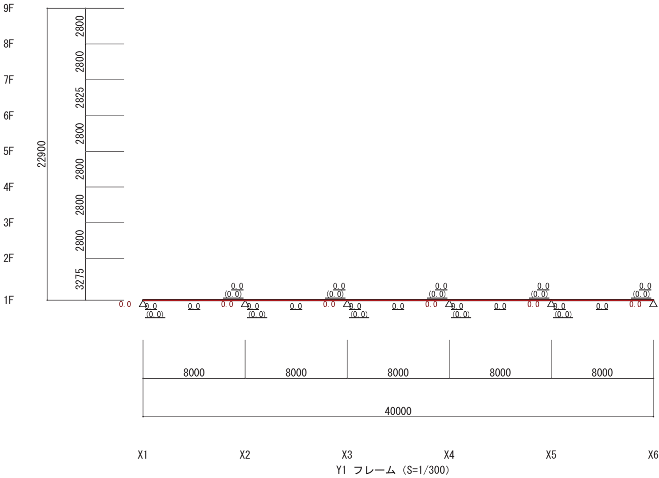
地震力(X方向 正加力) (立体解析)
