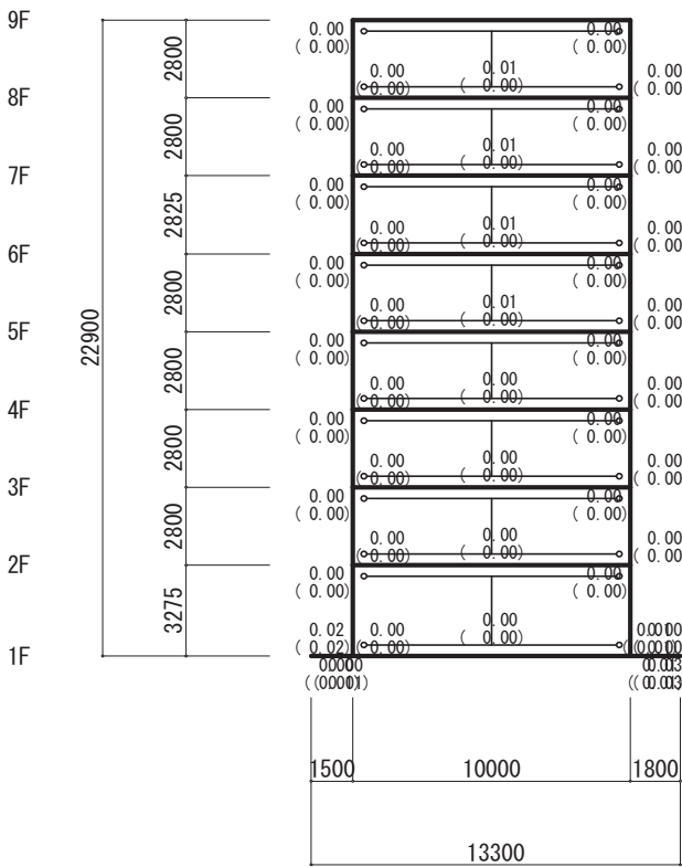
Y1 Y2 Y3 Y4 X1 フレーム (S=1/300)
