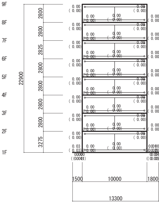
Y1 Y2 Y3 Y4 X3 フレーム (S=1/300)
