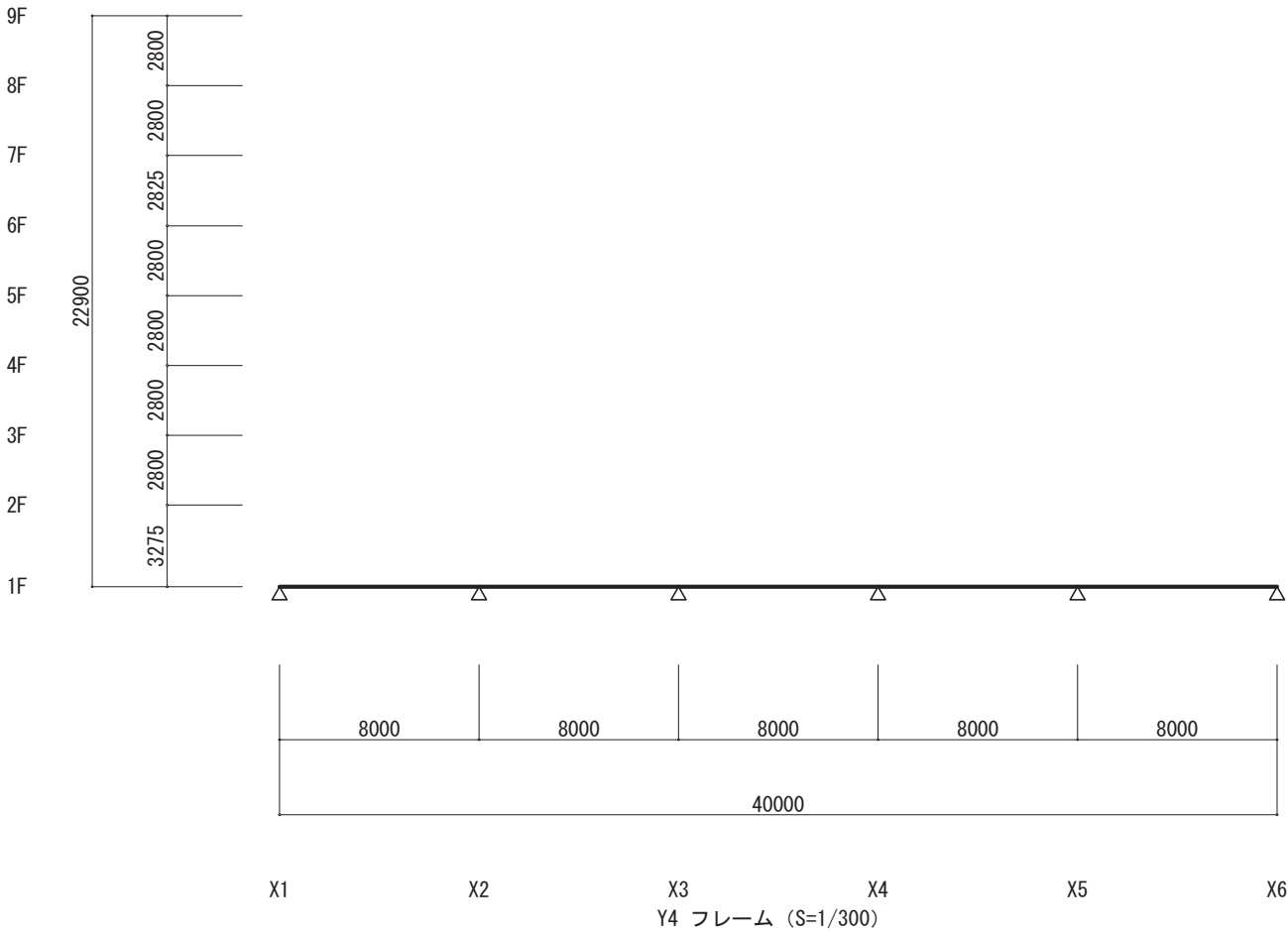
ヒンジ図（X方向 負加力）（立体MSモデル）（Ds算定時）
