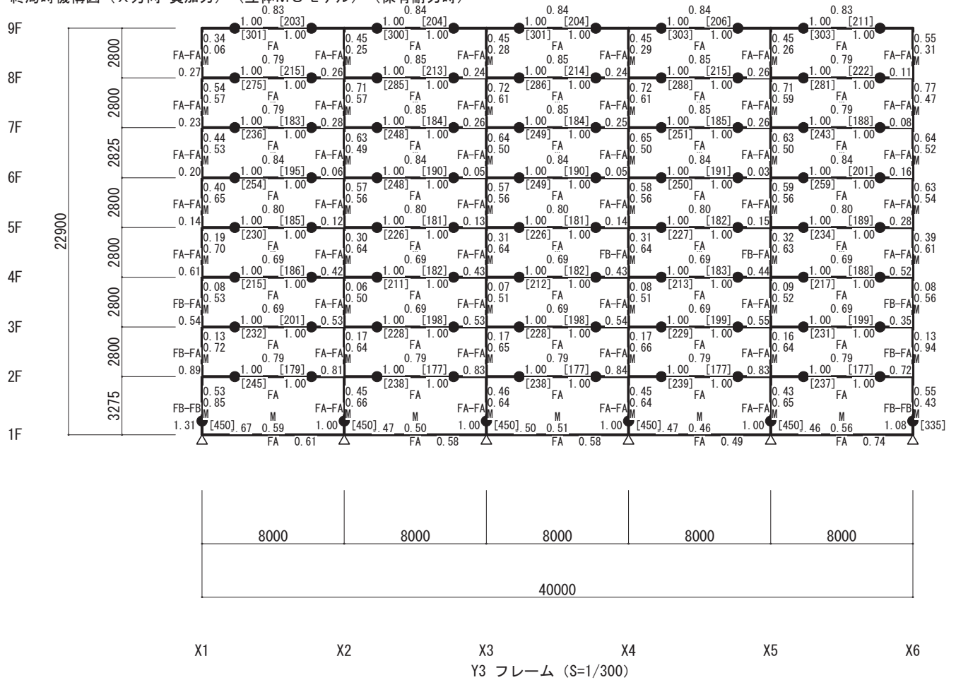
終局時機構図（X方向 負加力）（立体MSモデル）（保有耐力時）
