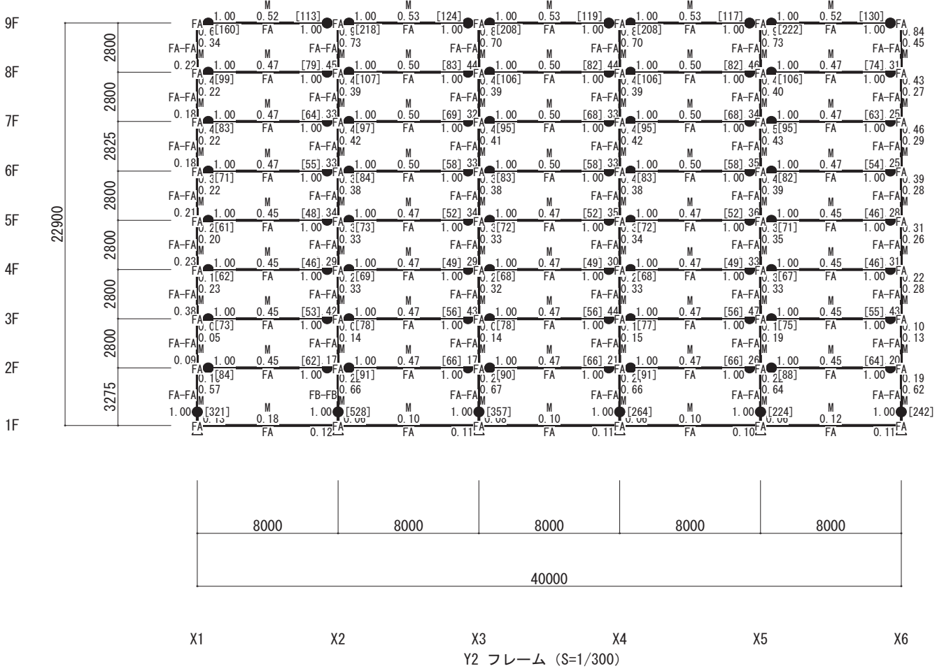
終局時機構図 (X方向 正加力) (立体MSモデル) (Ds算定時)
