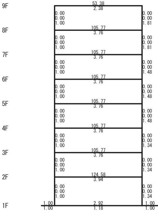
Y1 Y2 Y3 Y4 X3 フレーム (S=1/263)
