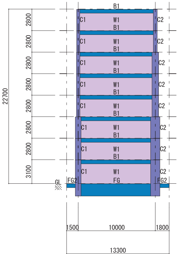
X1 X2 X3 X4 X5 X6 Y4 フレーム (S=1/300)
