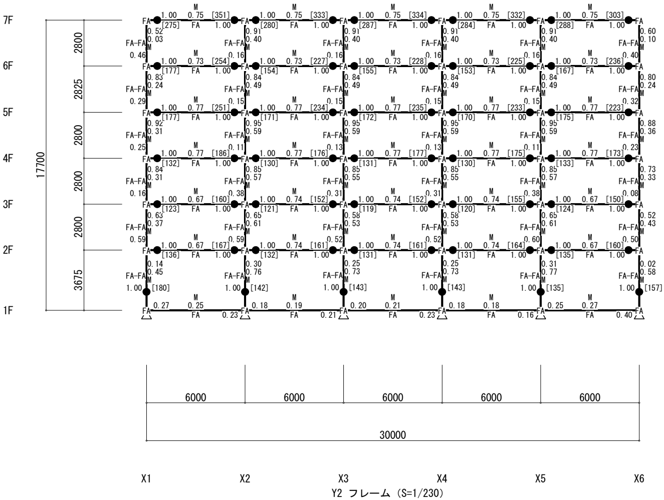
終局時機構図（X方向 正加力）（立体MSモデル）（Ds算定時）
