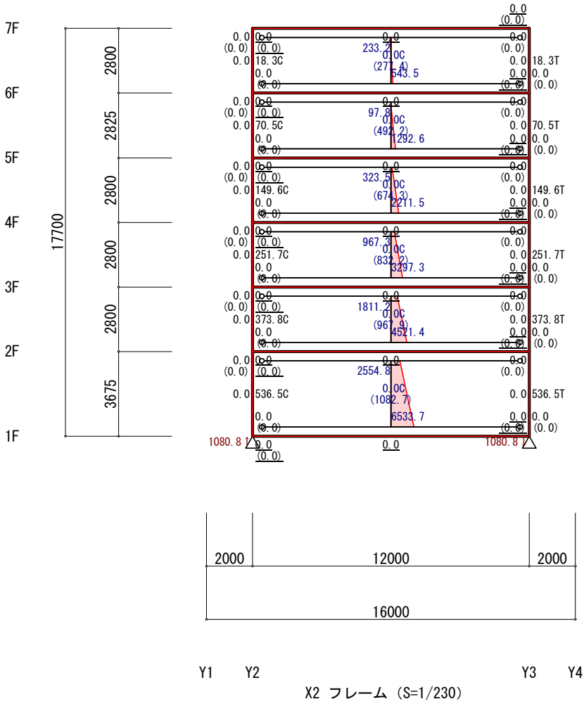
地震力(Y方向 負加力) (立体解析)
