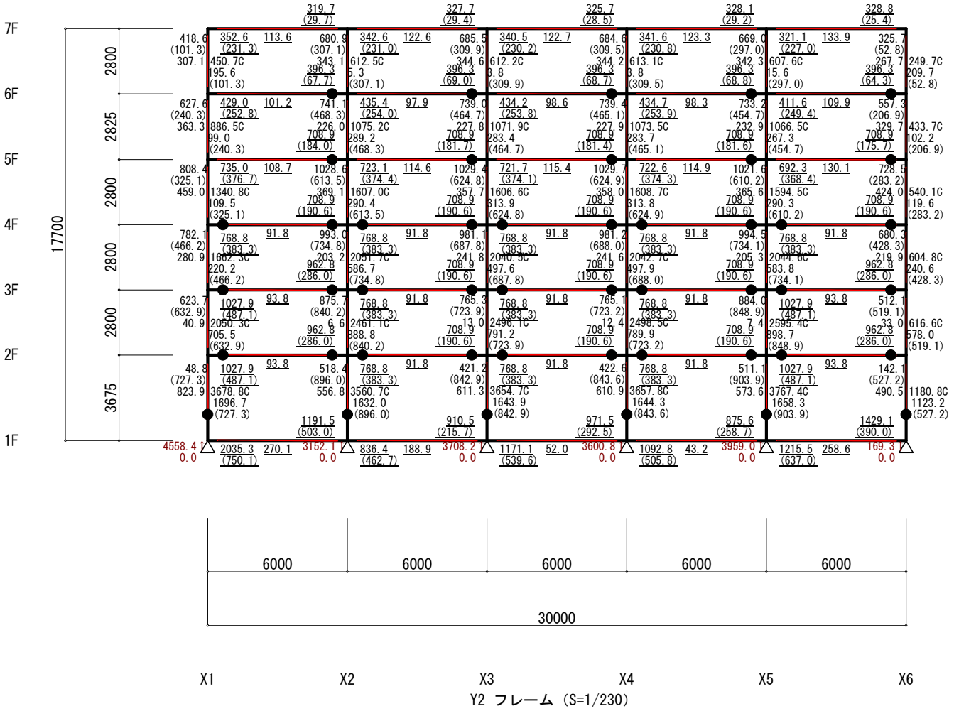
長期考慮危険断面位置応力（X方向 負加力）（立体MSモデル）（保有耐力時）
