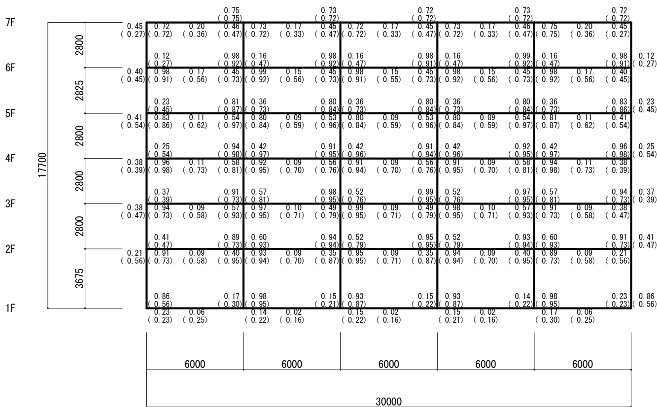
X1 X2 X3 X4 X5 X6 Y2 フレーム (S=1/230)
