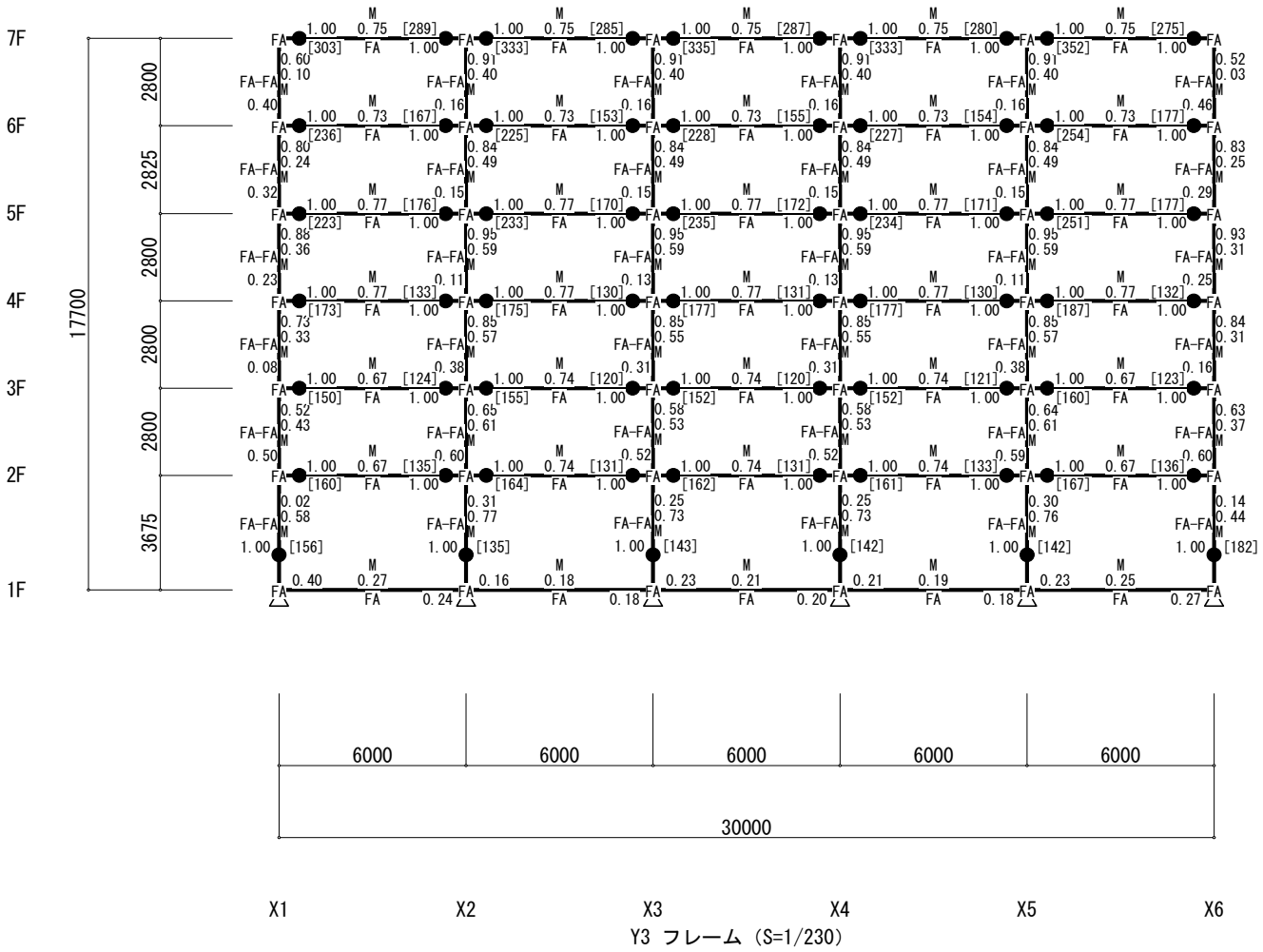
終局時機構図（X方向 負加力）（立体MSモデル）（Ds算定時）
