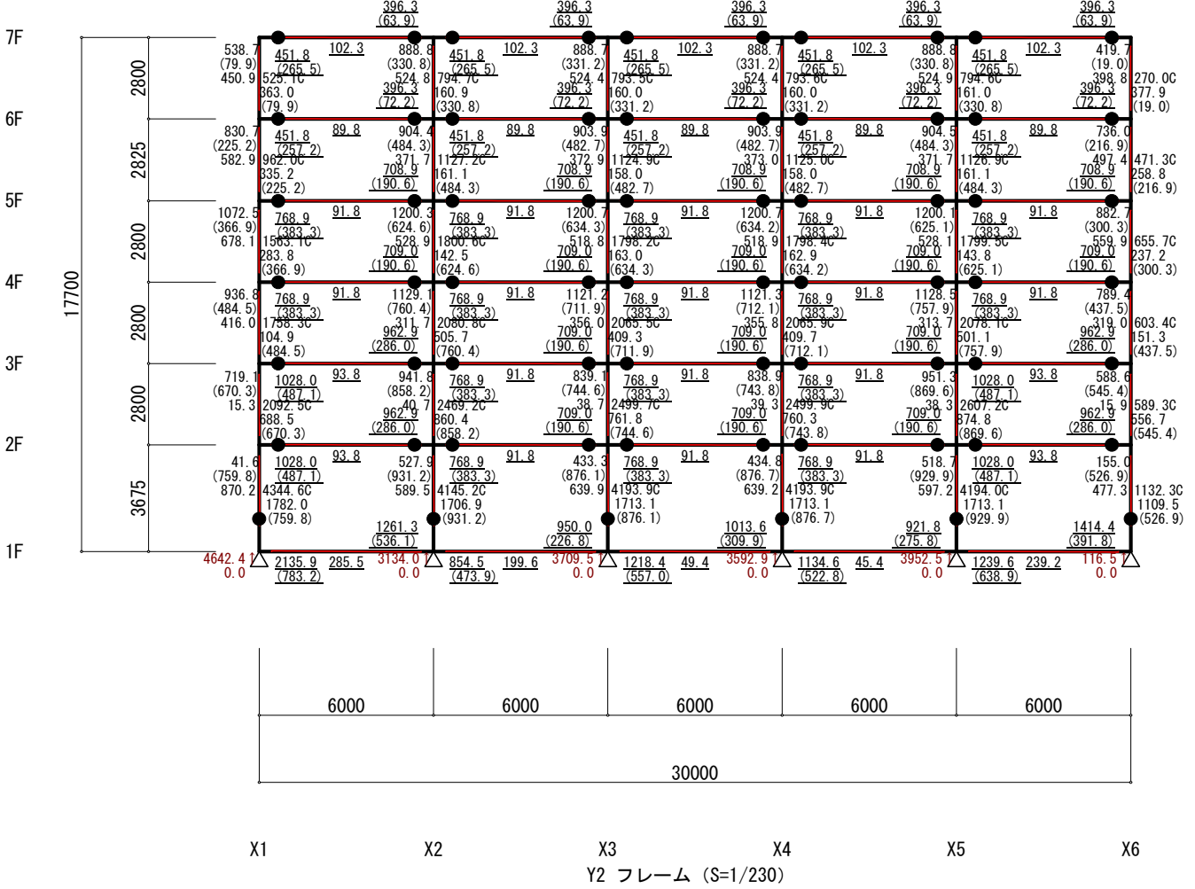
長期考慮危険断面位置応力（X方向 負加力）（立体MSモデル）（Ds算定時）
