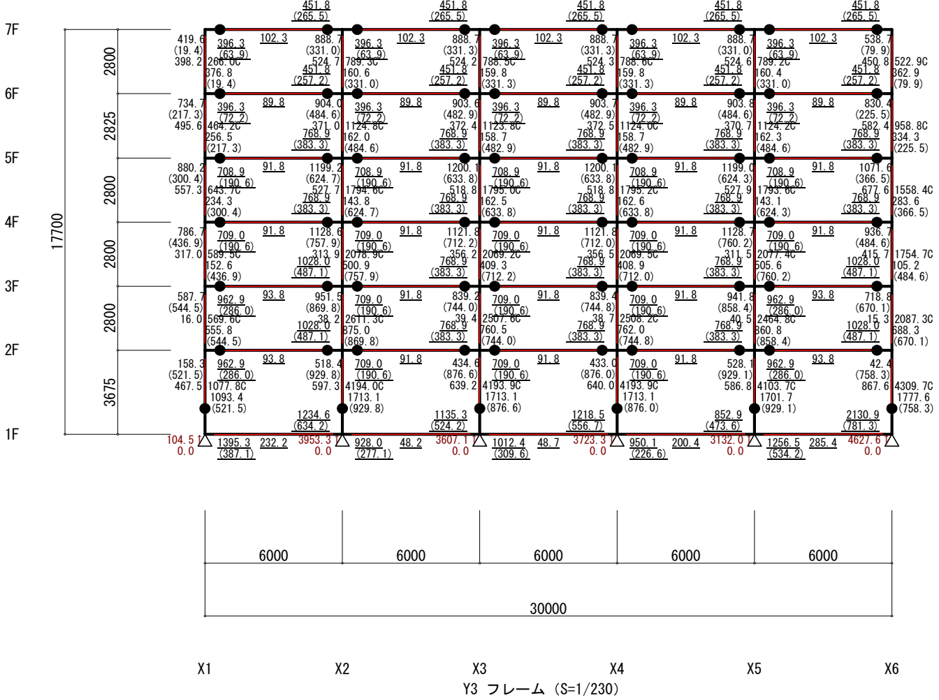
長期考慮危険断面位置応力（X方向 正加力）（立体MSモデル）（Ds算定時）
