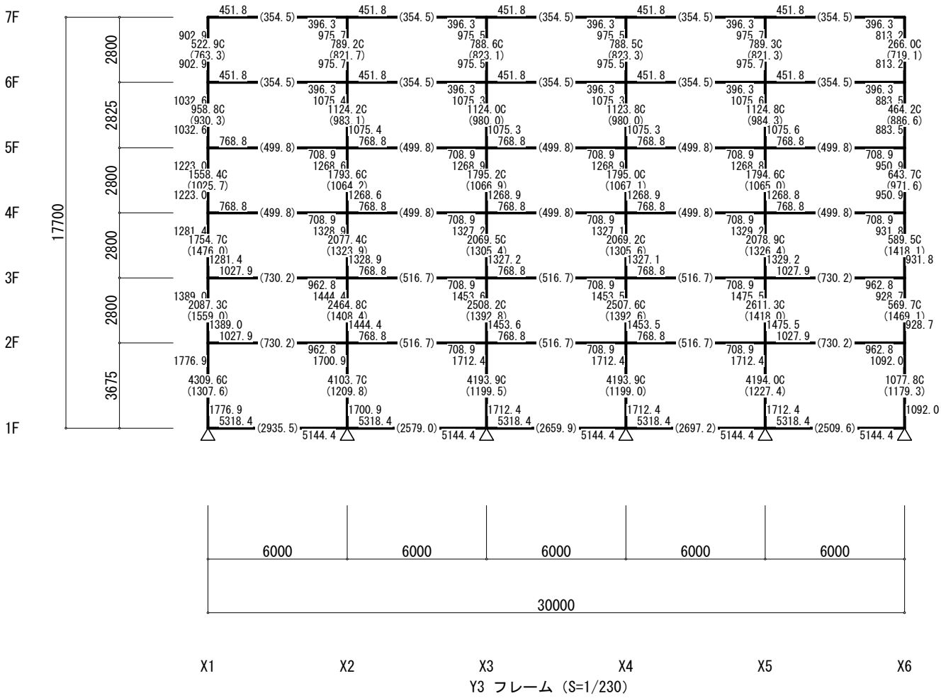
終局強度 (X方向 負加力) (立体MSモデル) (Ds算定時)
