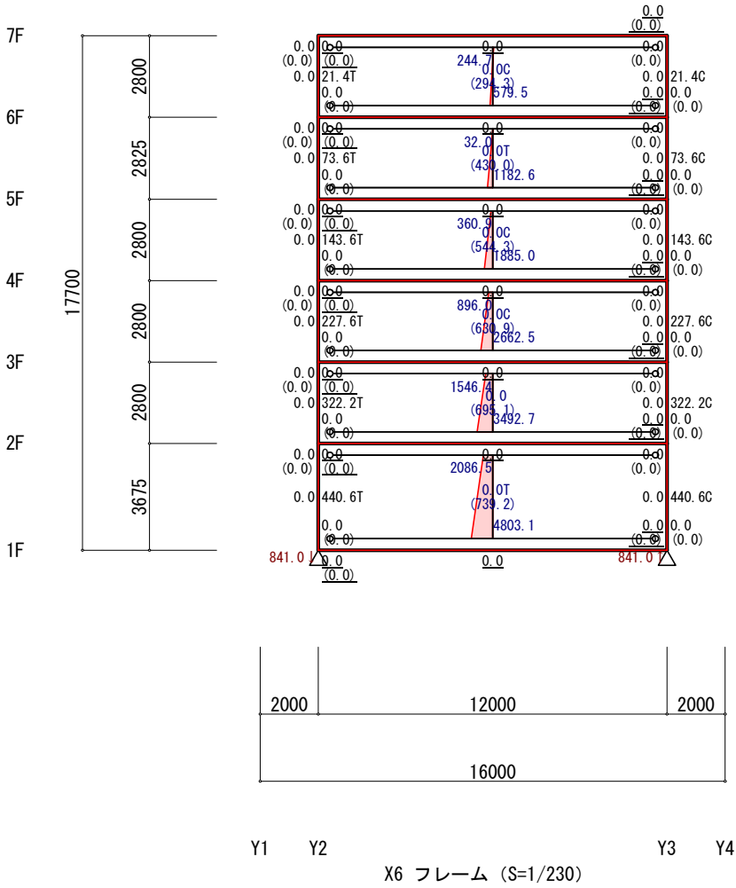
地震力(Y方向 正加力) (立体解析)
