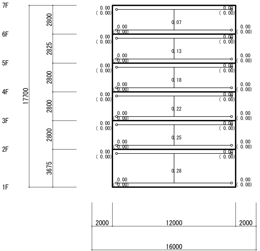
Y1 Y2 Y3 Y4 X2 フレーム (S=1/230)
