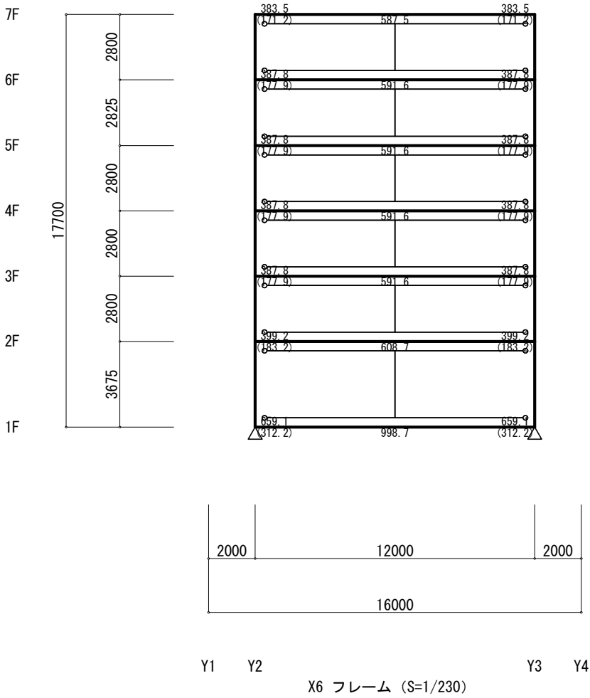
固定荷重+積載荷重
