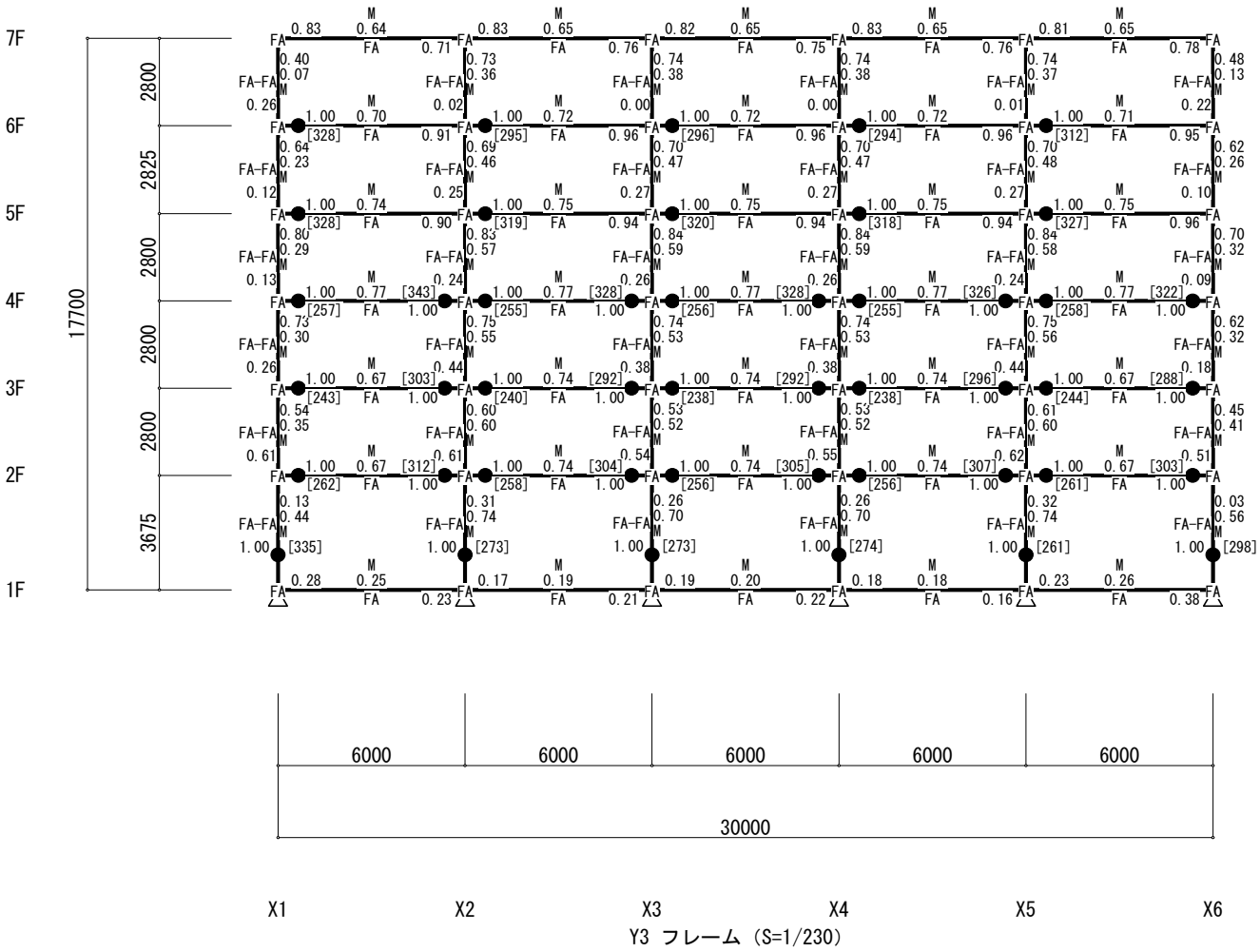
終局時機構図（X方向 正加力）（立体MSモデル）（保有耐力時）
