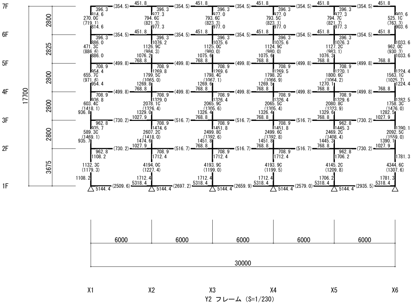
終局強度 (X方向 正加力) (立体MSモデル) (Ds算定時)
