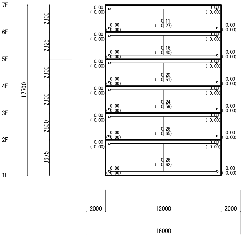
Y1 Y2 X6 フレーム (S=1/230) Y3 Y4
