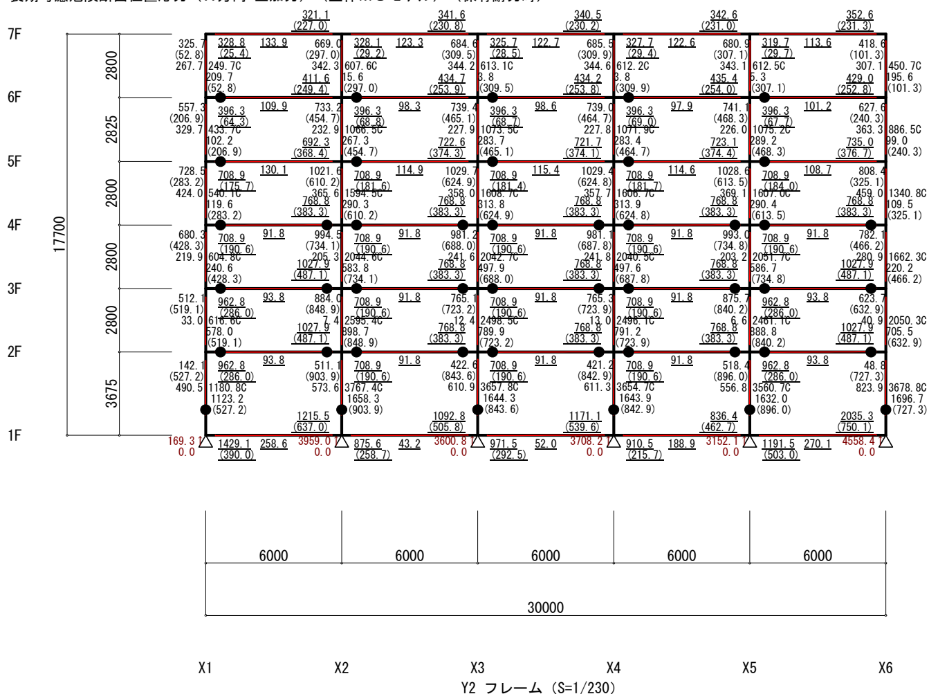
長期考慮危険断面位置応力 (X方向 正加力) (立体MSモデル) (保有耐力時)
