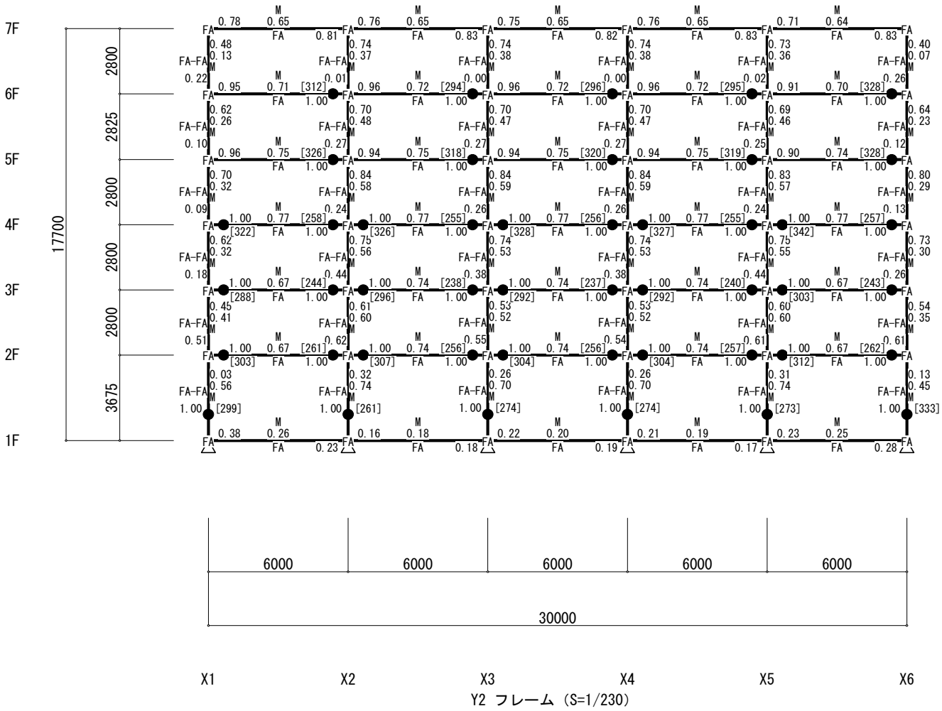
終局時機構図（X方向 負加力）（立体MSモデル）（保有耐力時）
