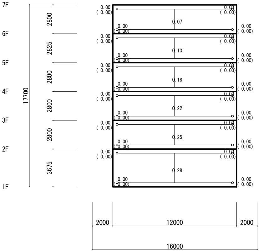
Y1 Y2 X5 フレーム (S=1/230) Y3 Y4
