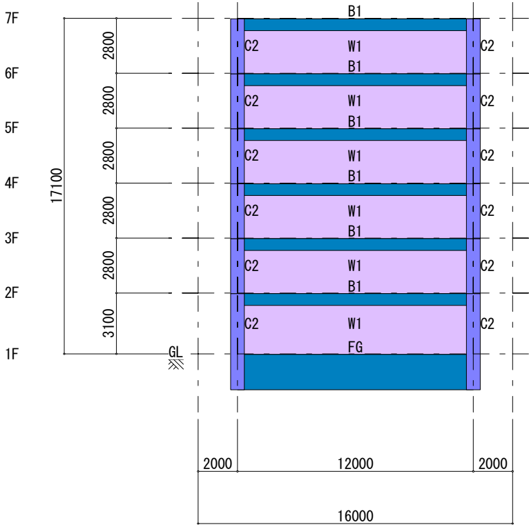
Y1 Y2 Y3 Y4 X3 フレーム (S=1/265)
