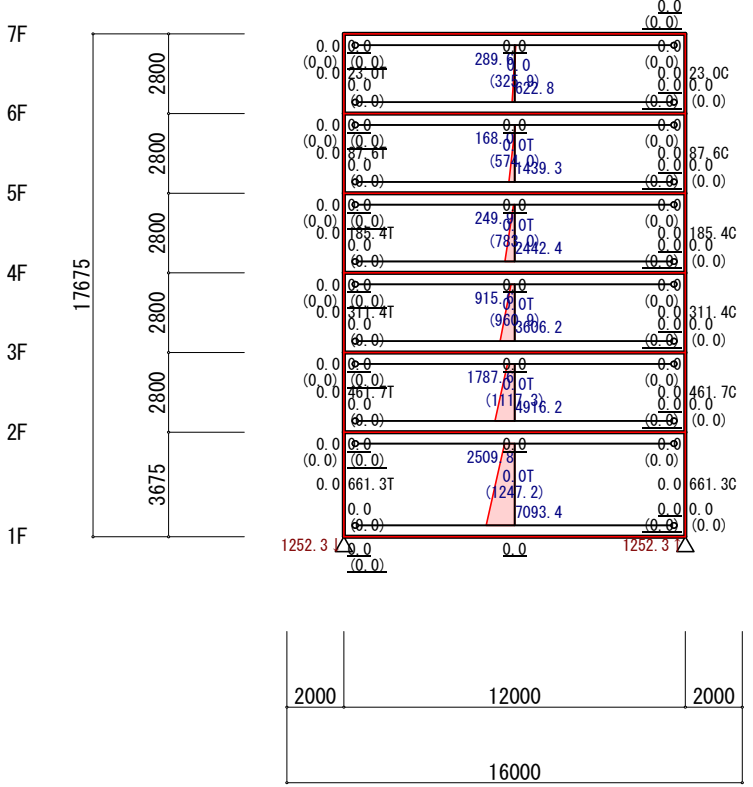
地震力(Y方向 正加力) (立体解析)
