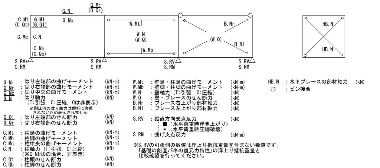
水平荷重時節点応力（X方向 正加力）（立体MSモデル）（保有耐力時）
