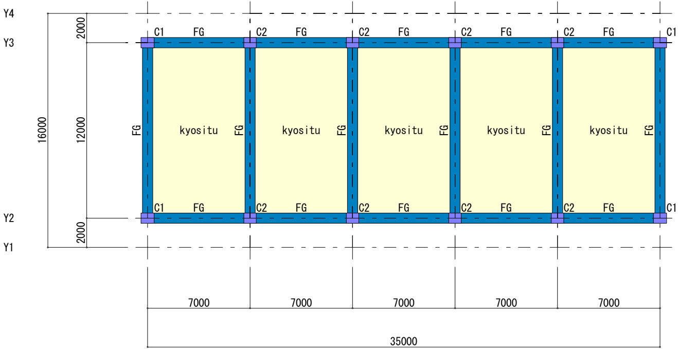
2F 層 (S=1/265)
