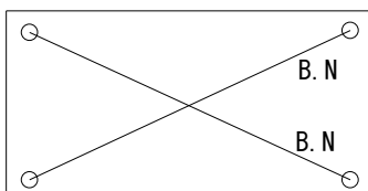
終局強度 (X方向 正加力) (立体MSモデル) (Ds算定時)
