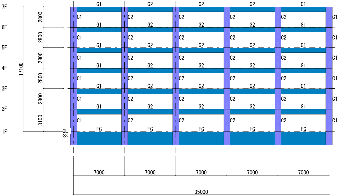
X1 X2 X3 X4 X5 X6 Y3 フレーム (S=1/265)
