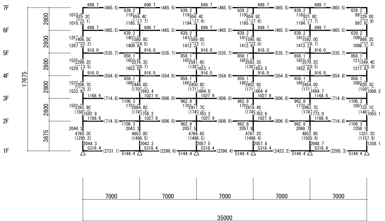
終局強度 (X方向 負加力) (立体MSモデル) (Ds算定時)
