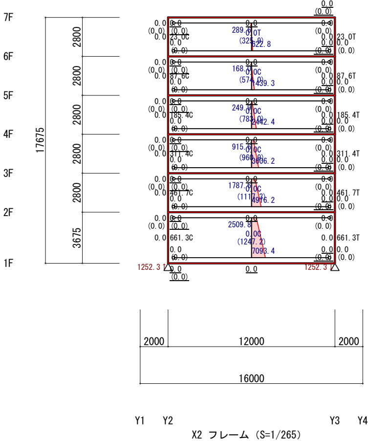
地震力(Y方向 負加力) (立体解析)
