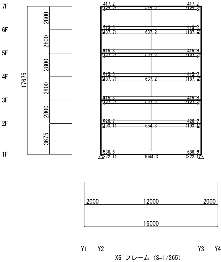
固定荷重+積載荷重
