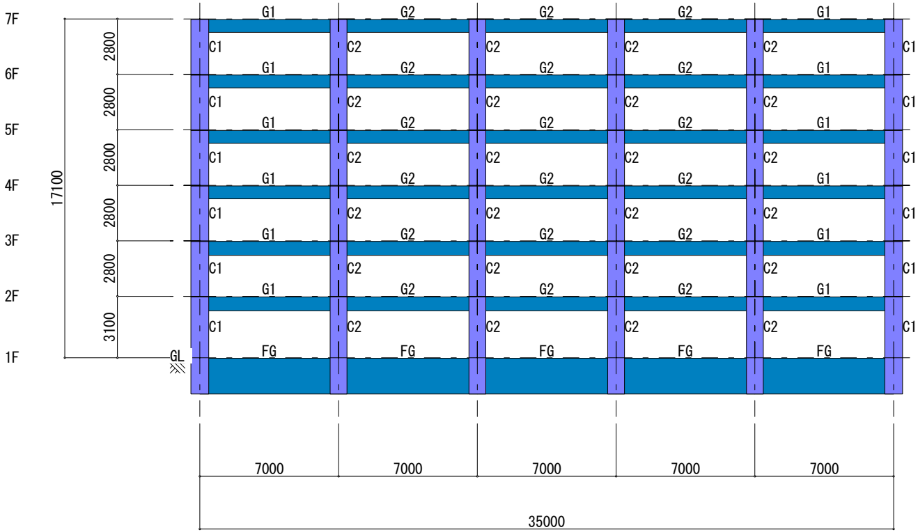
X1 X2 X3 X4 X5 X6 Y2 フレーム (S=1/265)
