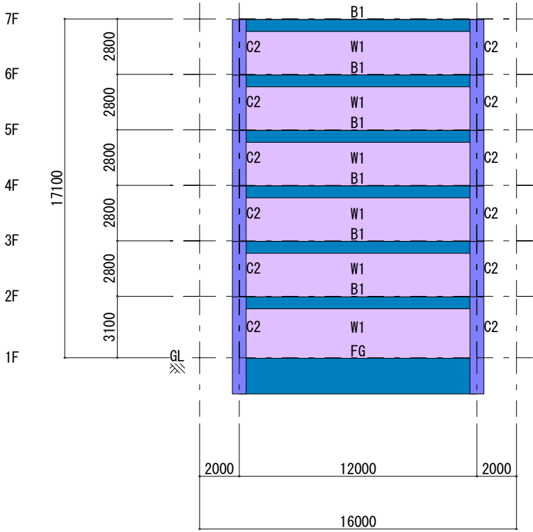
Y1 Y2 Y3 Y4 X2 フレーム (S=1/265)
