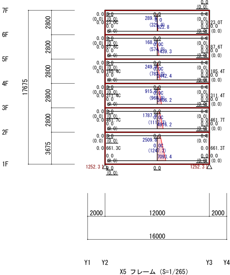
地震力(Y方向 負加力) (立体解析)
