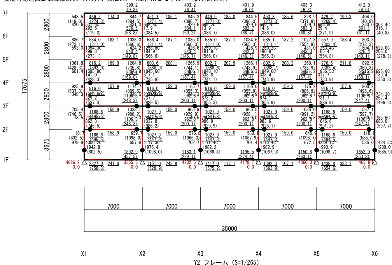
長期考慮危険断面位置応力 (X方向 負加力) (立体MSモデル) (保有耐力時)
