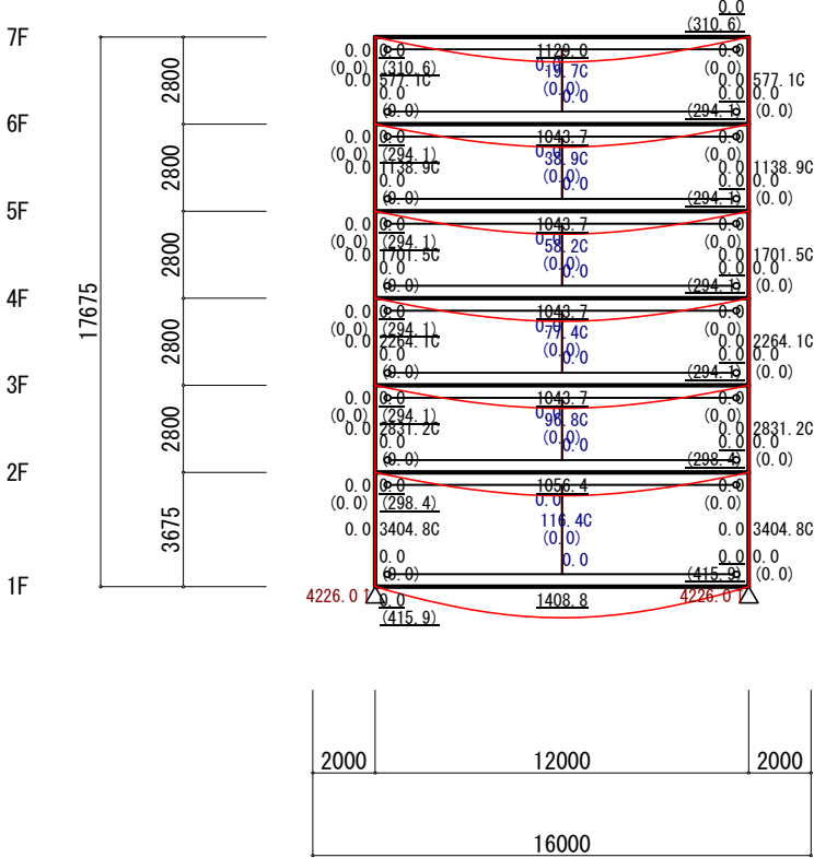
鉛直荷重 (立体解析)
