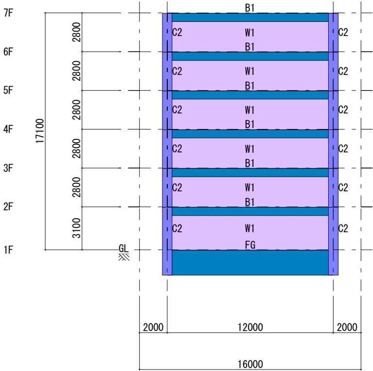
Y1 Y2 Y3 Y4 X5 フレーム (S=1/265)
