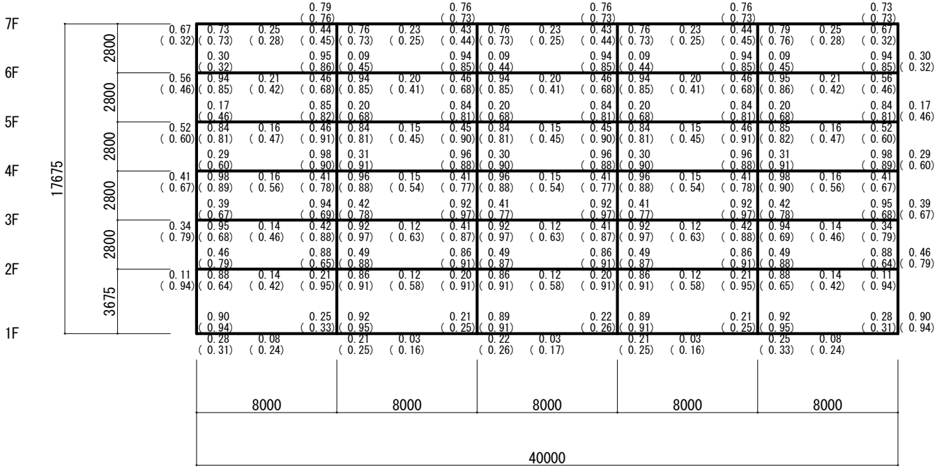
X1 X2 X3 X4 X5 X6 Y3 フレーム (S=1/300)
