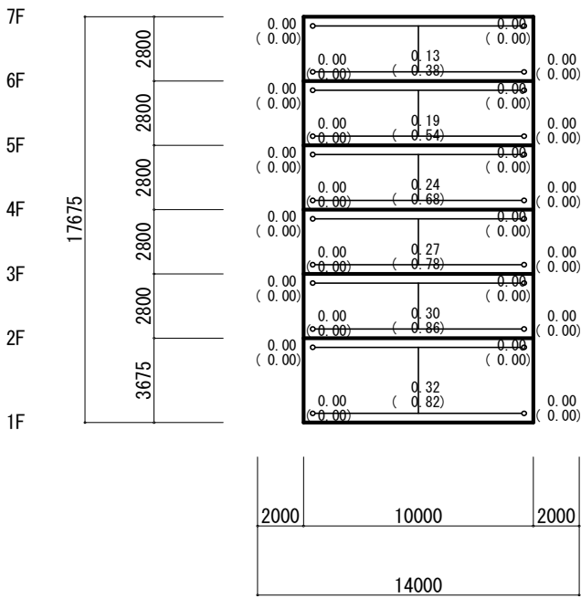
Y1 Y2 Y3 Y4 X6 フレーム (S=1/300)
