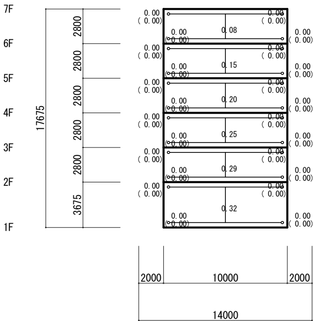
Y1 Y2 Y3 Y4 X5 フレーム (S=1/300)
