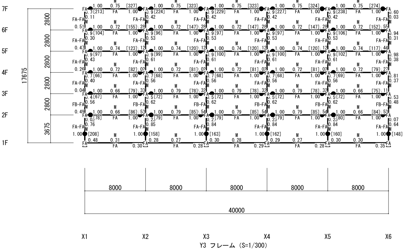
終局時機構図（X方向 負加力）（立体MSモデル）（Ds算定時）
