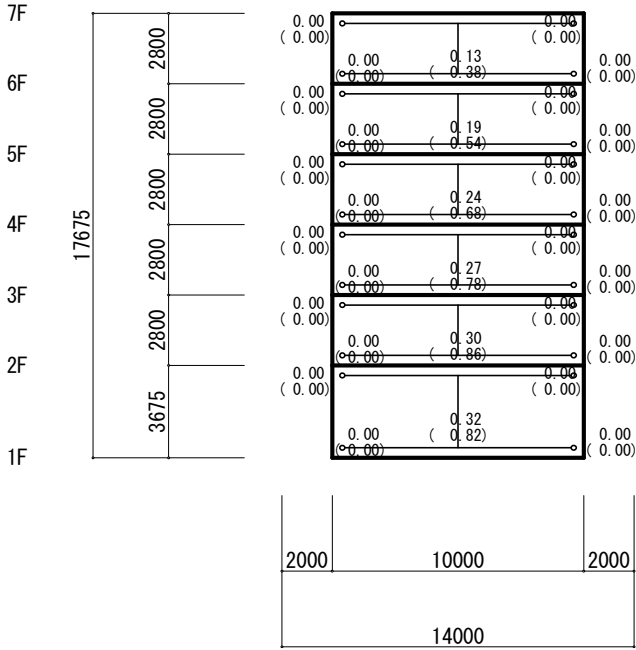
Y1 Y2 Y3 Y4 X1 フレーム (S=1/300)
