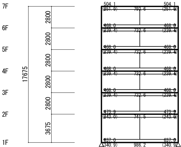
固定荷重+積載荷重
