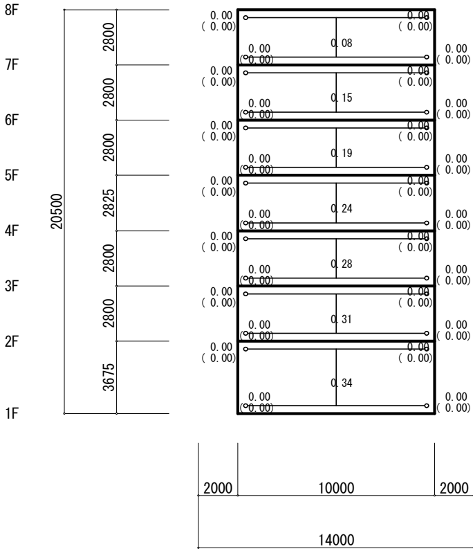
Y1 Y2 Y3 Y4 X4 フレーム (S=1/265)
