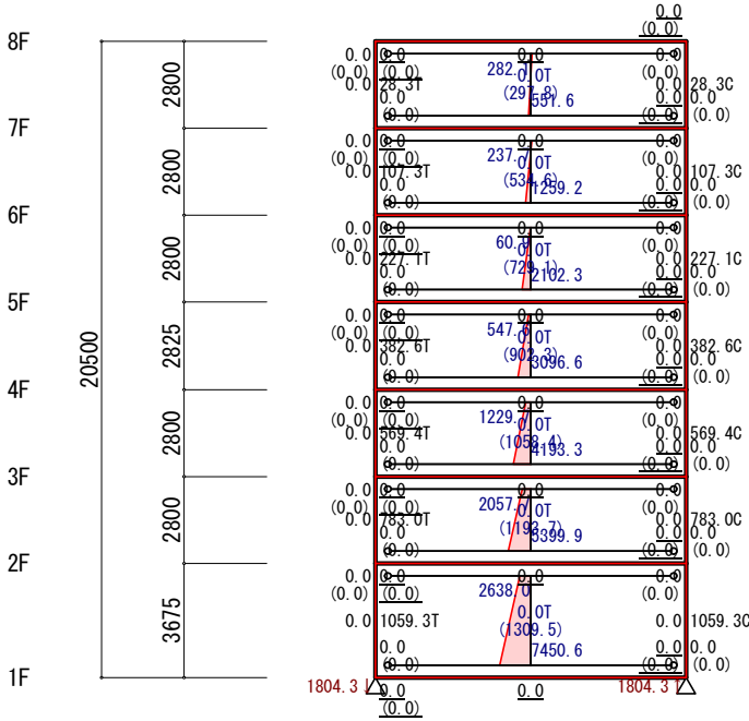
地震力(Y方向 正加力) (立体解析)
