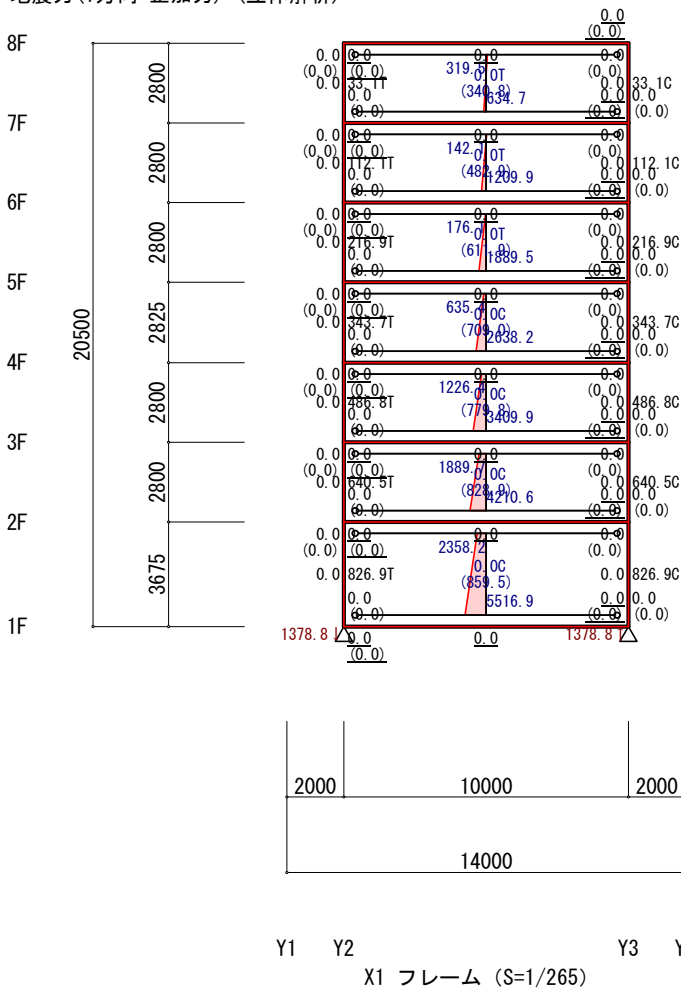
地震力 (Y方向 正加力) (立体解析)
