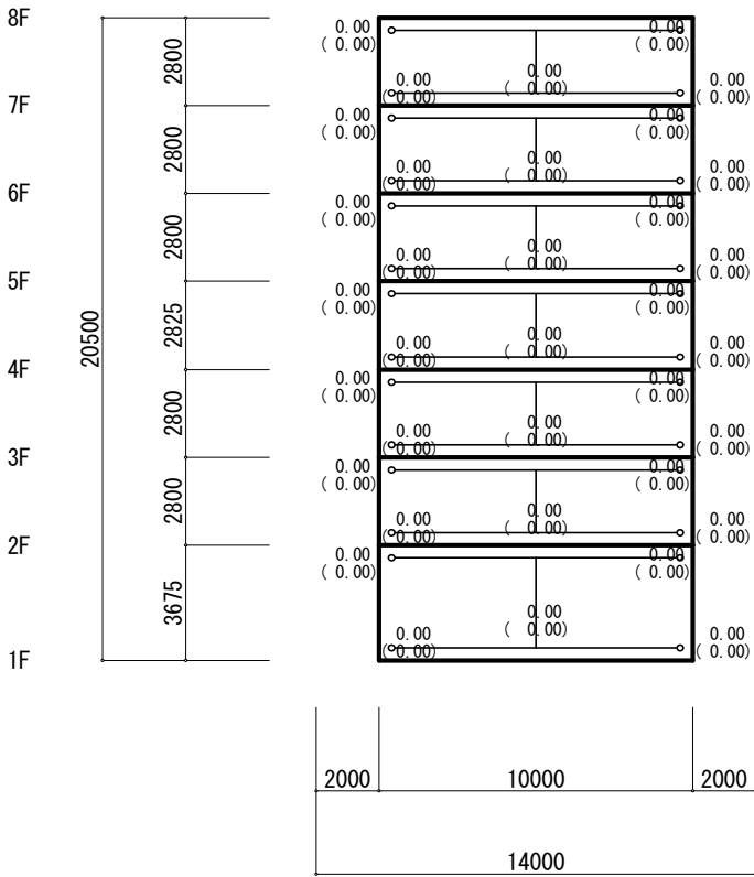
Y1 Y2 Y3 Y4 X6 フレーム (S=1/265)
