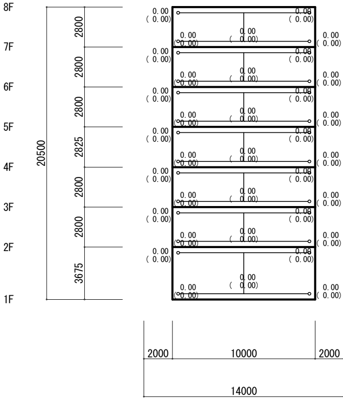
Y1 Y2 Y3 Y4 X2 フレーム (S=1/265)
