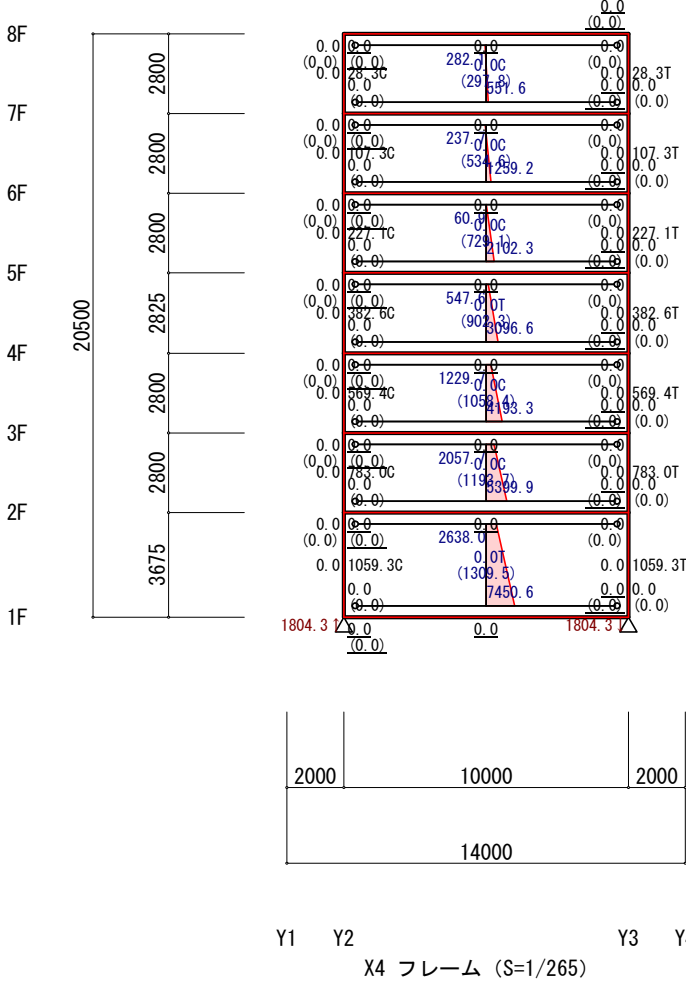
地震力 (Y方向 負加力) (立体解析)
