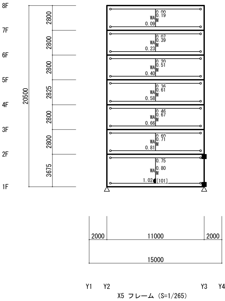
終局時機構図（Y方向 負加力）（立体MSモデル）（Ds算定時）
