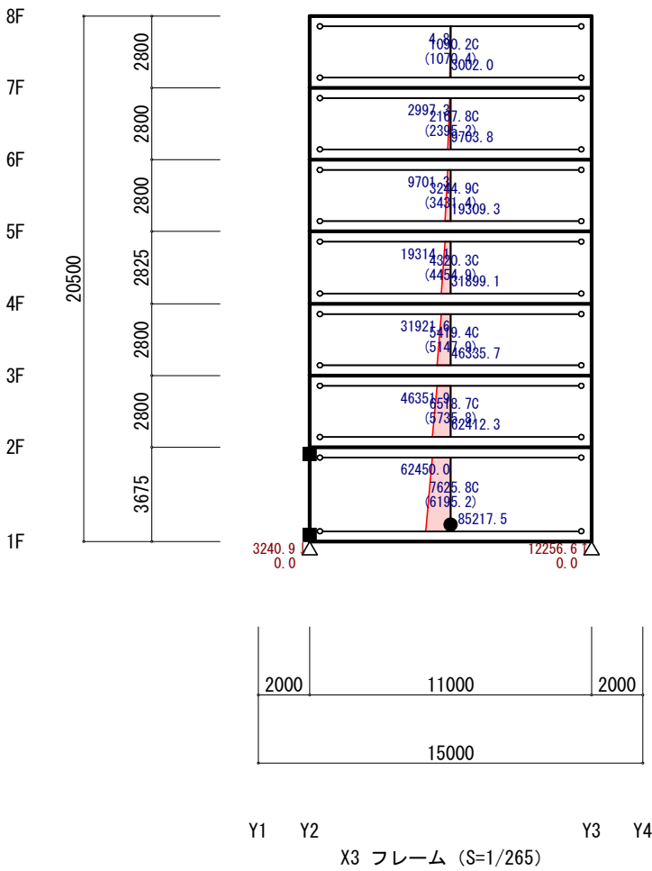
長期考慮危険断面位置応力（Y方向 正加力）（立体MSモデル）（保有耐力時）
