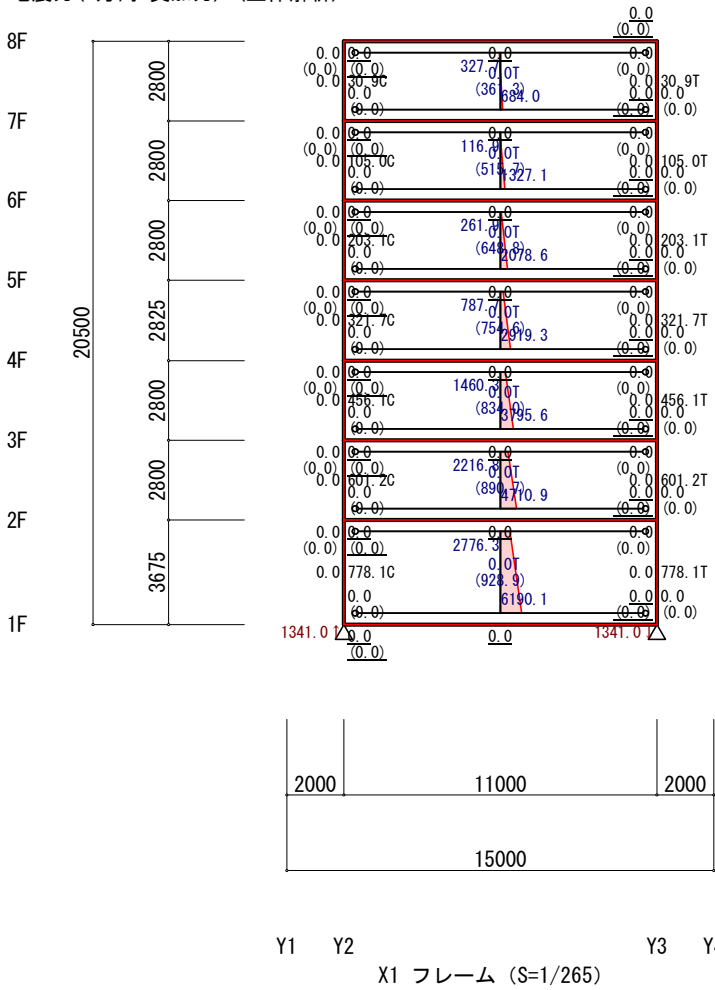
地震力 (Y方向 負加力) (立体解析)
