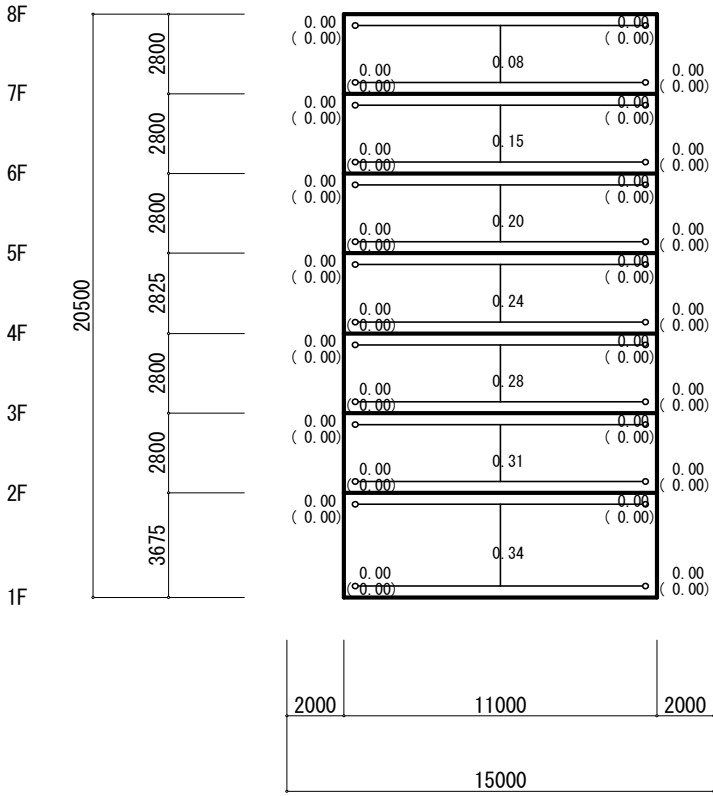
Y1 Y2 Y3 Y4 X4 フレーム (S=1/265)
