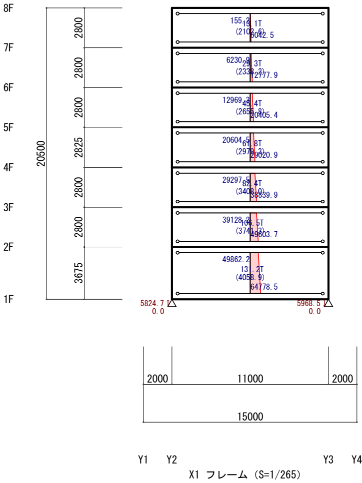
水平荷重時節点応力（Y方向 負加力）（立体MSモデル）（Ds算定時）
