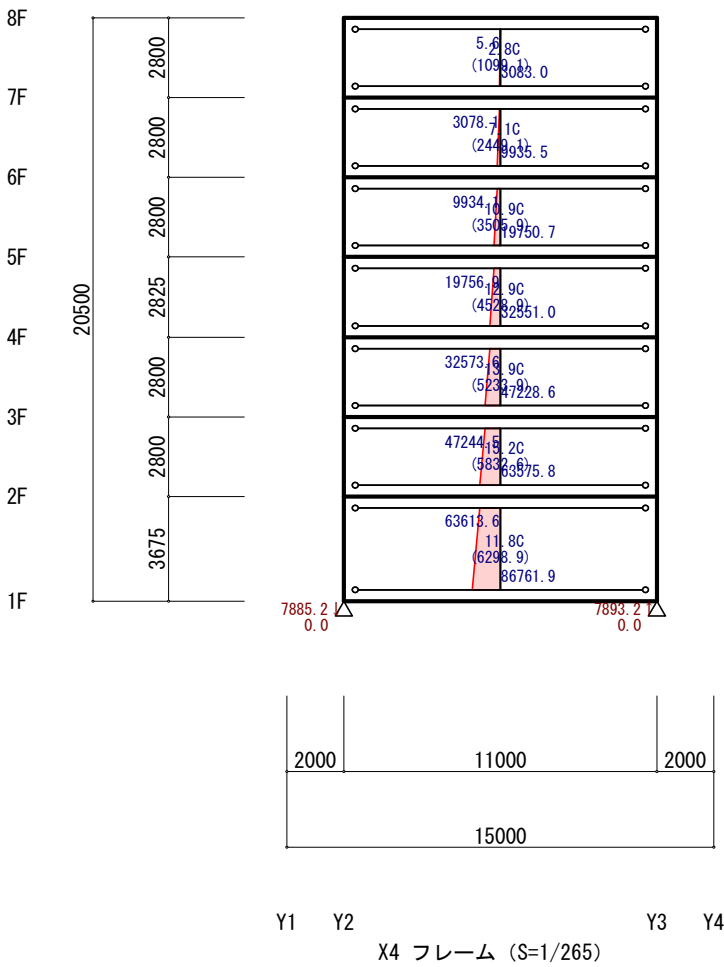
水平荷重時節点応力（Y方向 正加力）（立体MSモデル）（Ds算定時）
