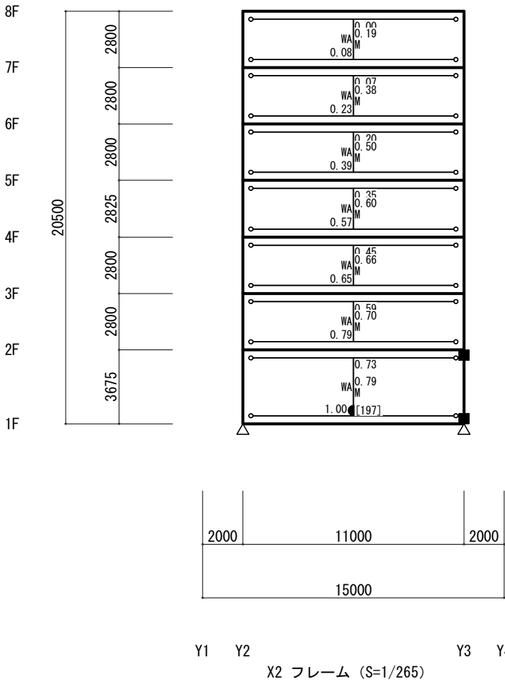
終局時機構図（Y方向 負加力）（立体MSモデル）（保有耐力時）
