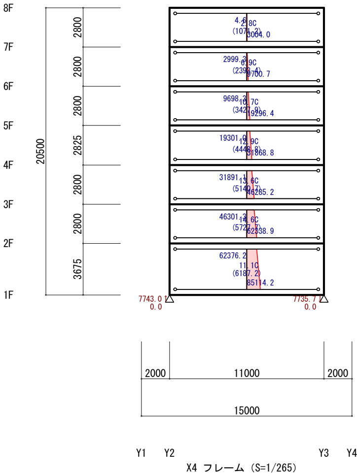
水平荷重時節点応力（Y方向 負加力）（立体MSモデル）（保有耐力時）
