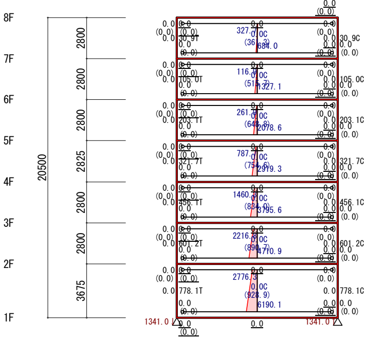
地震力(Y方向 正加力) (立体解析)
