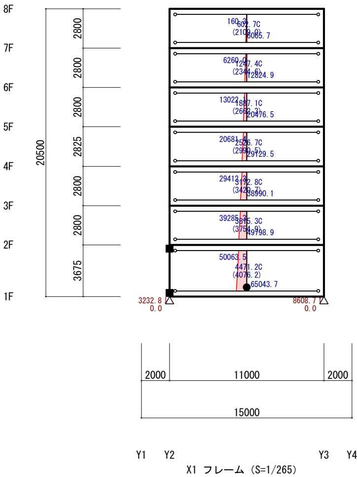
長期考慮危険断面位置応力（Y方向 正加力）（立体MSモデル）（Ds算定時）
