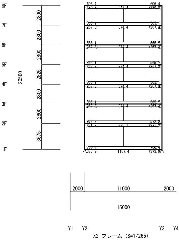
固定荷重+積載荷重
