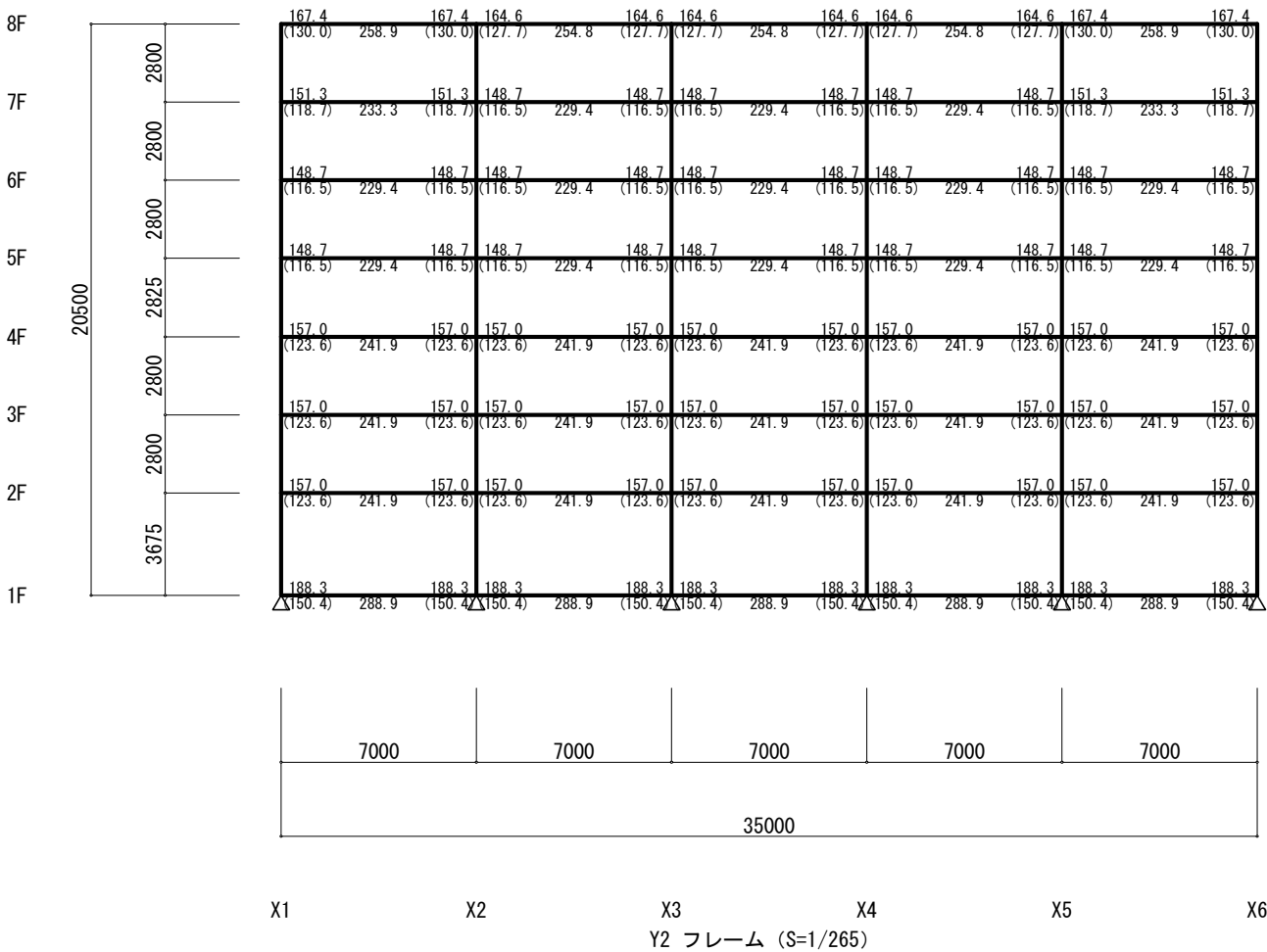
固定荷重+積載荷重
