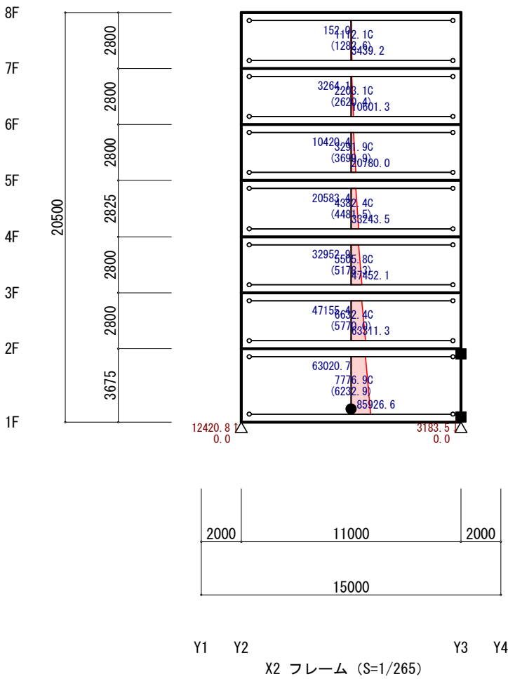
長期考慮危険断面位置応力（Y方向 負加力）（立体MSモデル）（保有耐力時）
