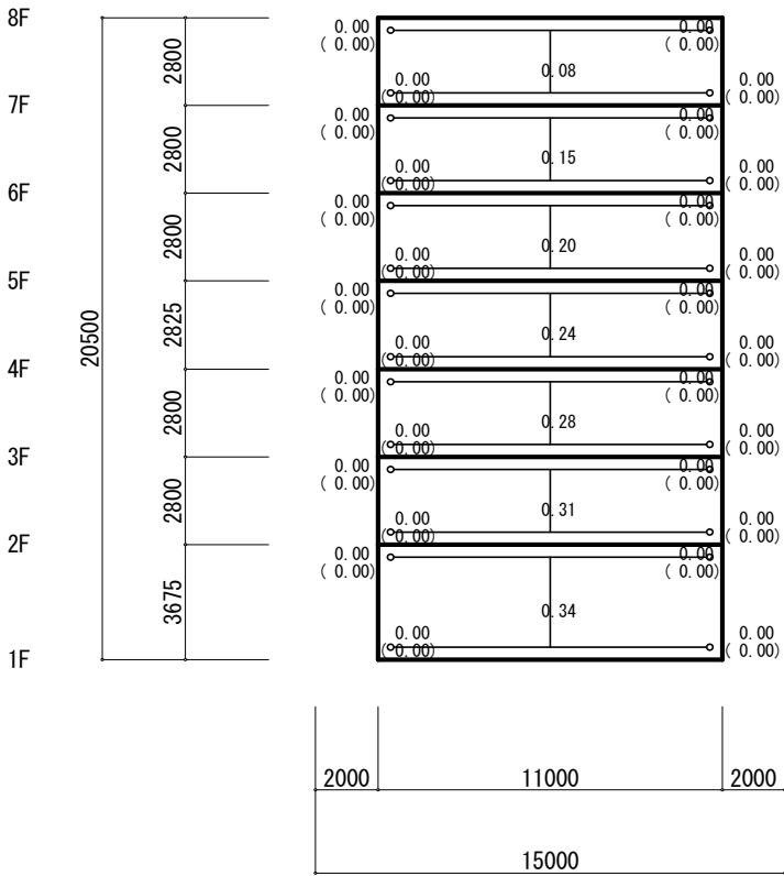
Y1 Y2 Y3 Y4 X5 フレーム (S=1/265)
