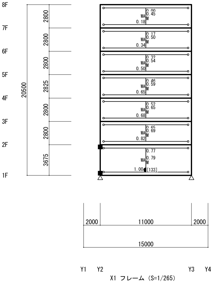
終局時機構図（Y方向 正加力）（立体MSモデル）（保有耐力時）
