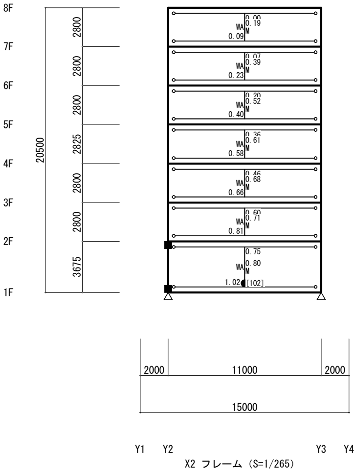
終局時機構図（Y方向 正加力）（立体MSモデル）（Ds算定時）
