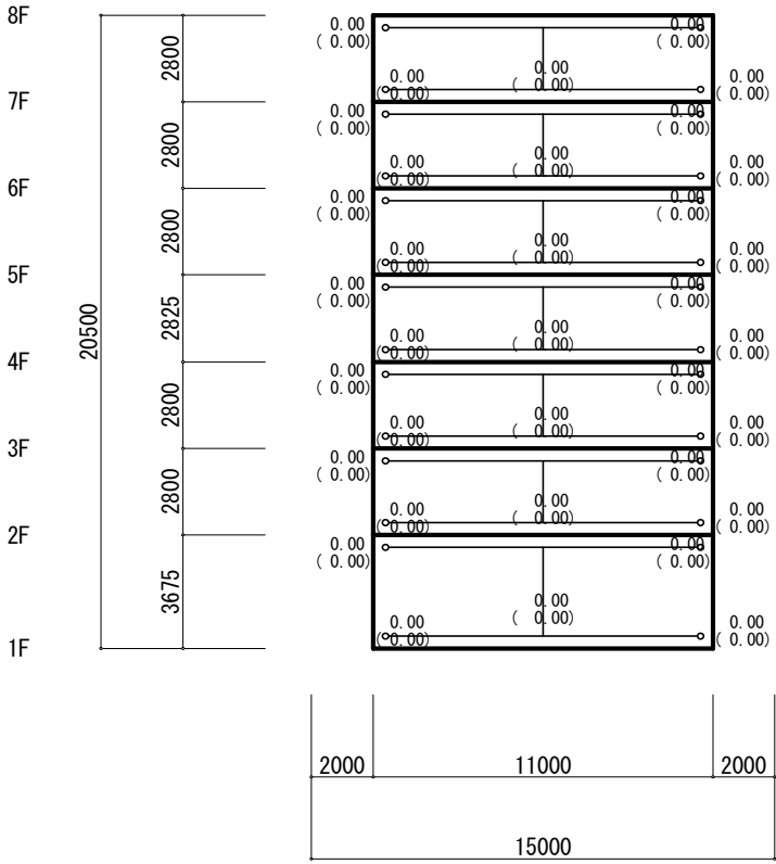
Y1 Y2 Y3 Y4 X2 フレーム (S=1/265)
