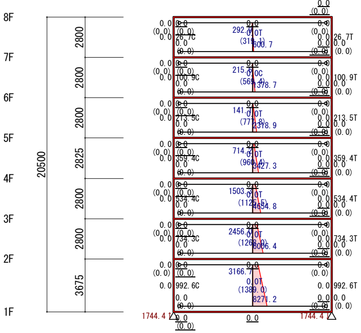
地震力 (Y方向 負加力) (立体解析)
