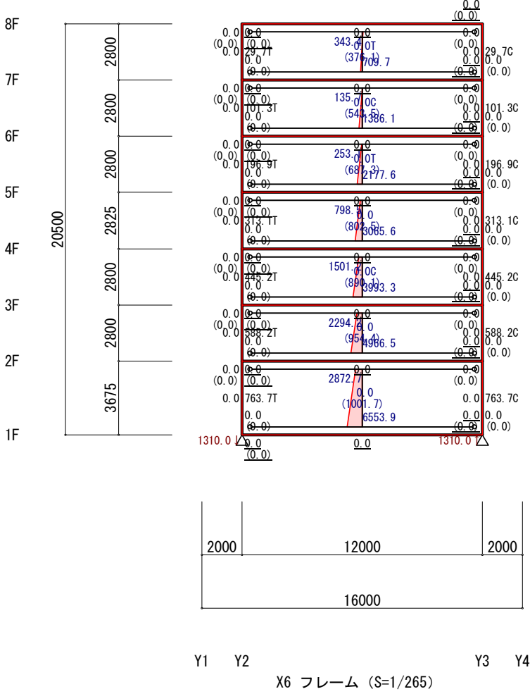
地震力 (Y方向 正加力) (立体解析)
