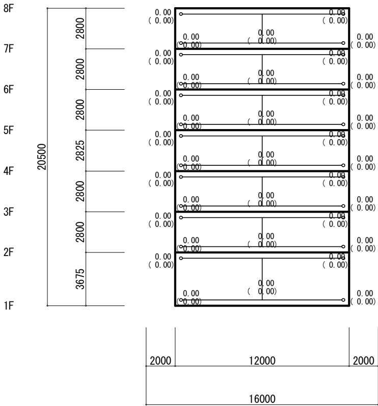
Y1 Y2 Y3 Y4 X5 フレーム (S=1/265)
