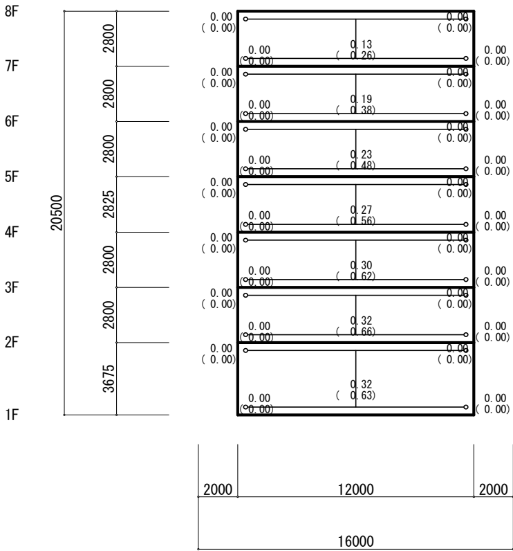
Y1 Y2 Y3 Y4 X1 フレーム (S=1/265)
