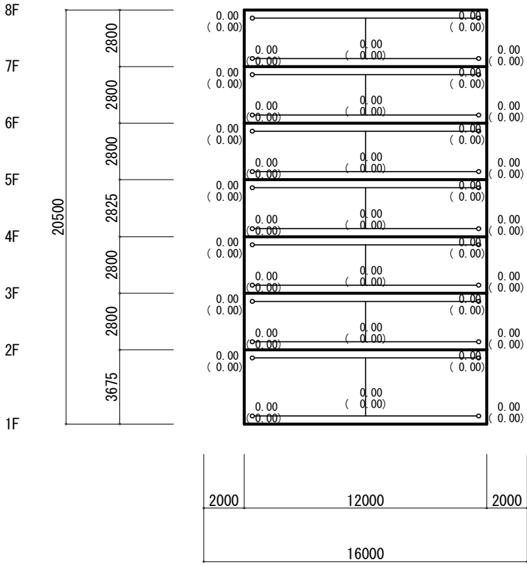
Y1 Y2 Y3 Y4 X6 フレーム (S=1/265)
