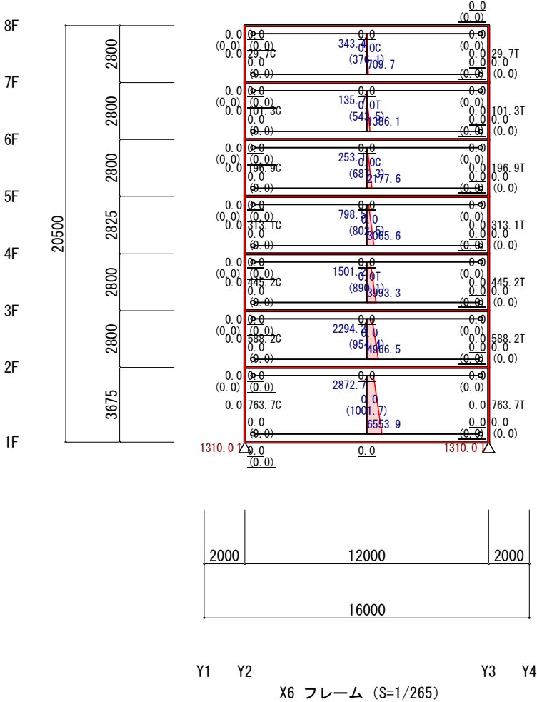
地震力(Y方向 負加力) (立体解析)
